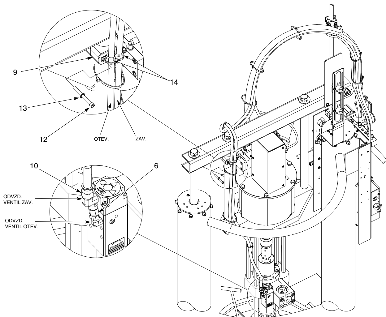
Obr. 14 55galonová černá hadice pro velký rám (pokr.)
