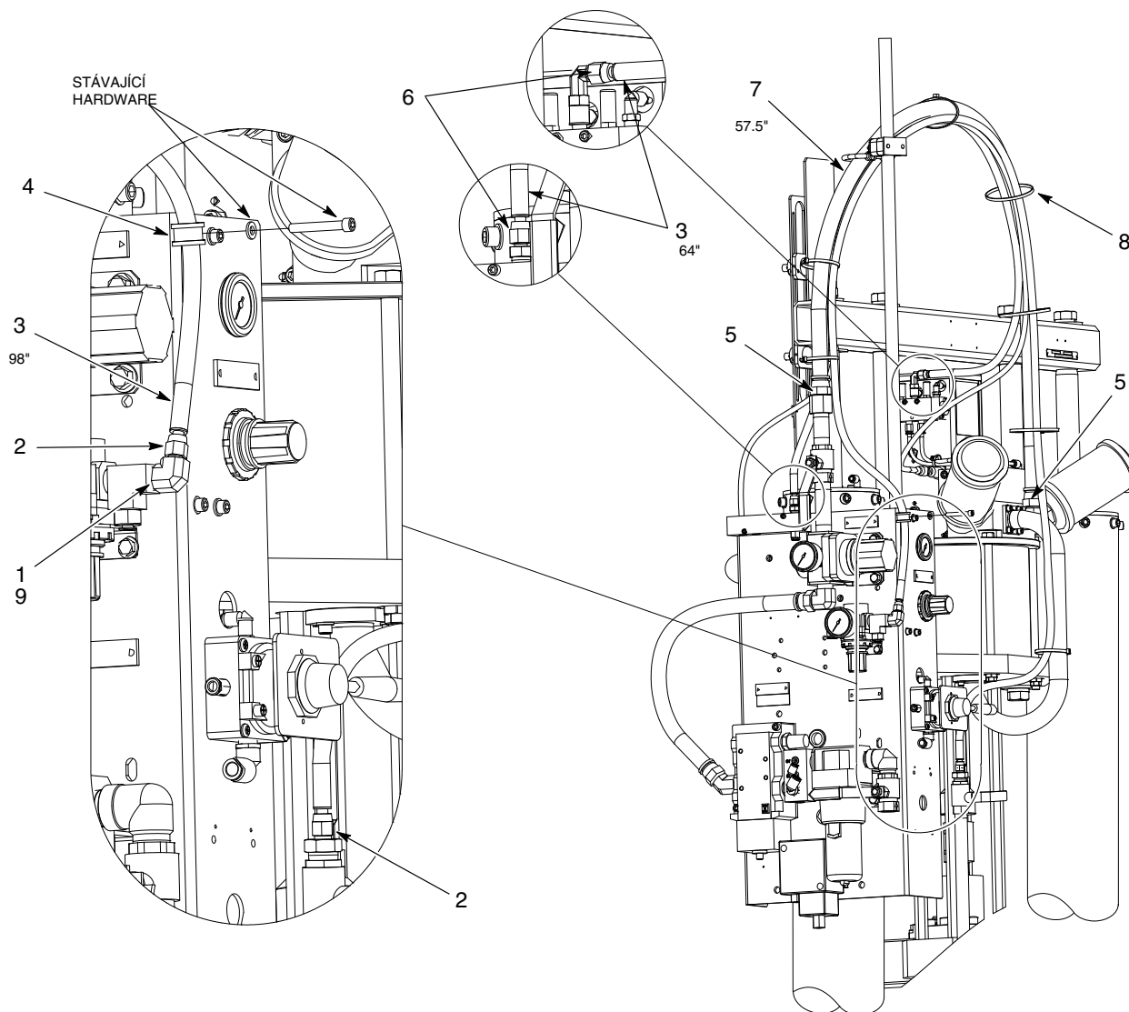
Obr. 4 5/30galonová žáruvzdorná hadice pro velký rám
