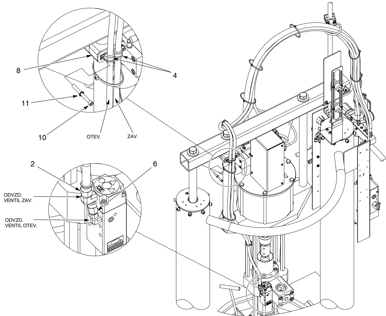
Obr. 7 5/30galonová žáruvzdorná hadice pro velký rám s odtlakováním (pokr.)
