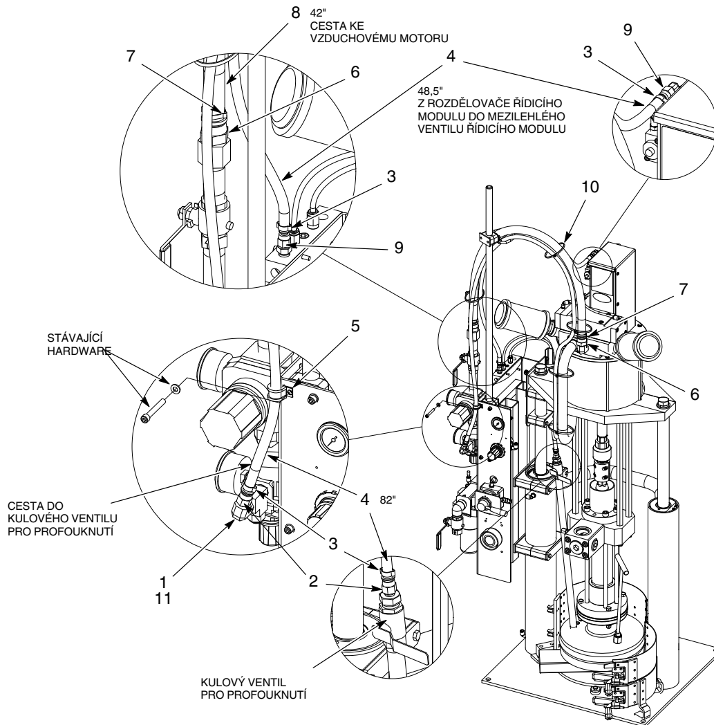
Obr. 3 Černá hadice pro malý rám
