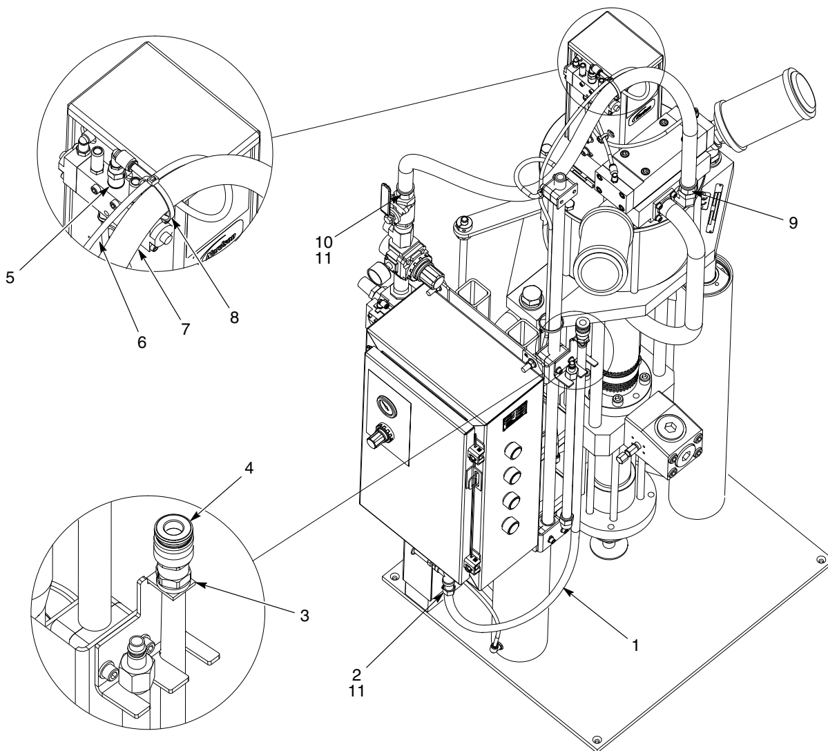
Obr. 18 Hadice pro malý rám CE Rhino VE
