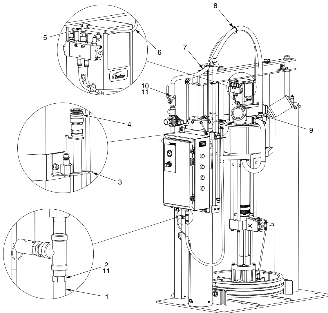
Obr. 20 Hadice pro velký rám CE Rhino VE
