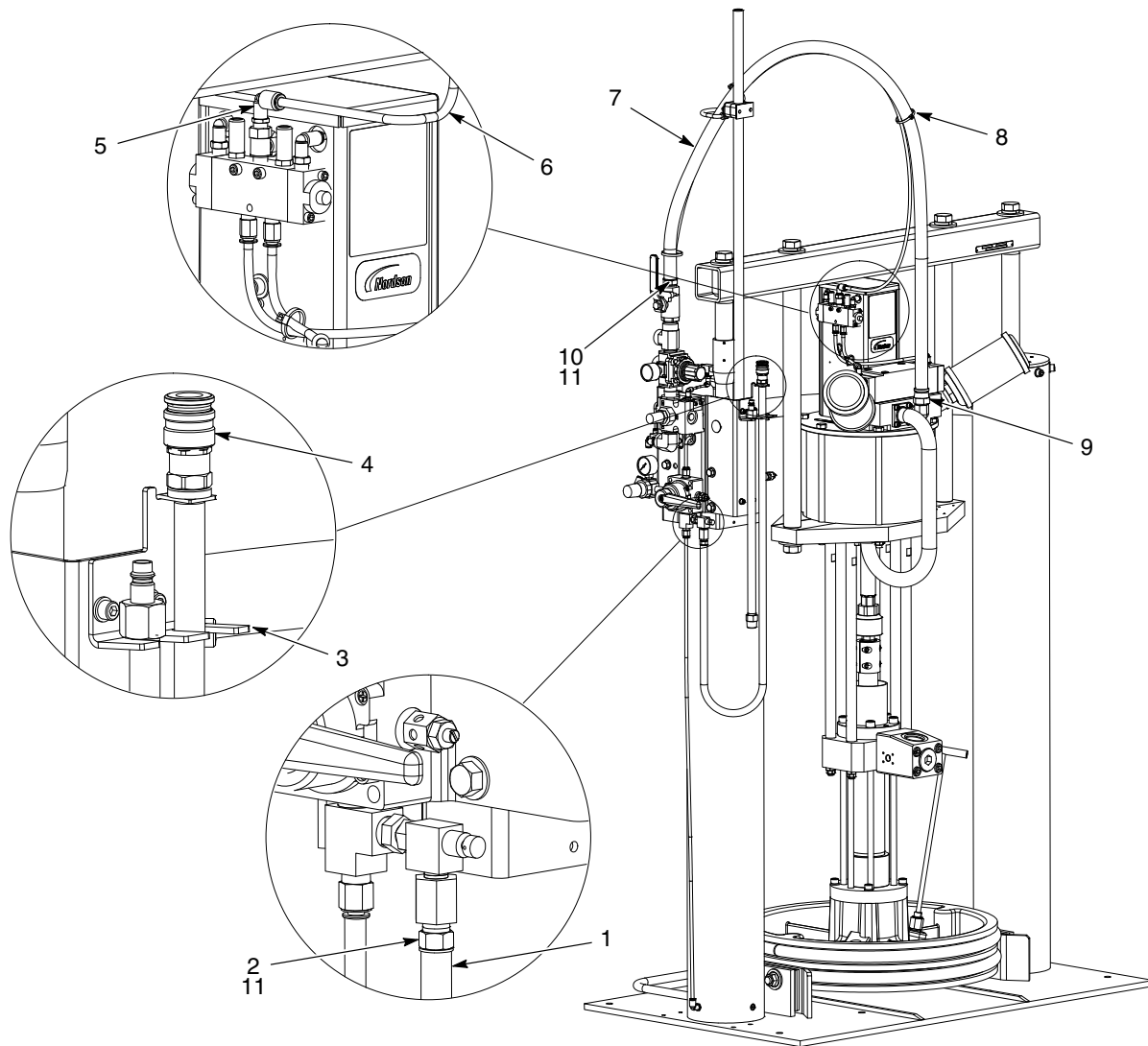
Obr. 19 Hadice pro velký rám CE Rhino VE
