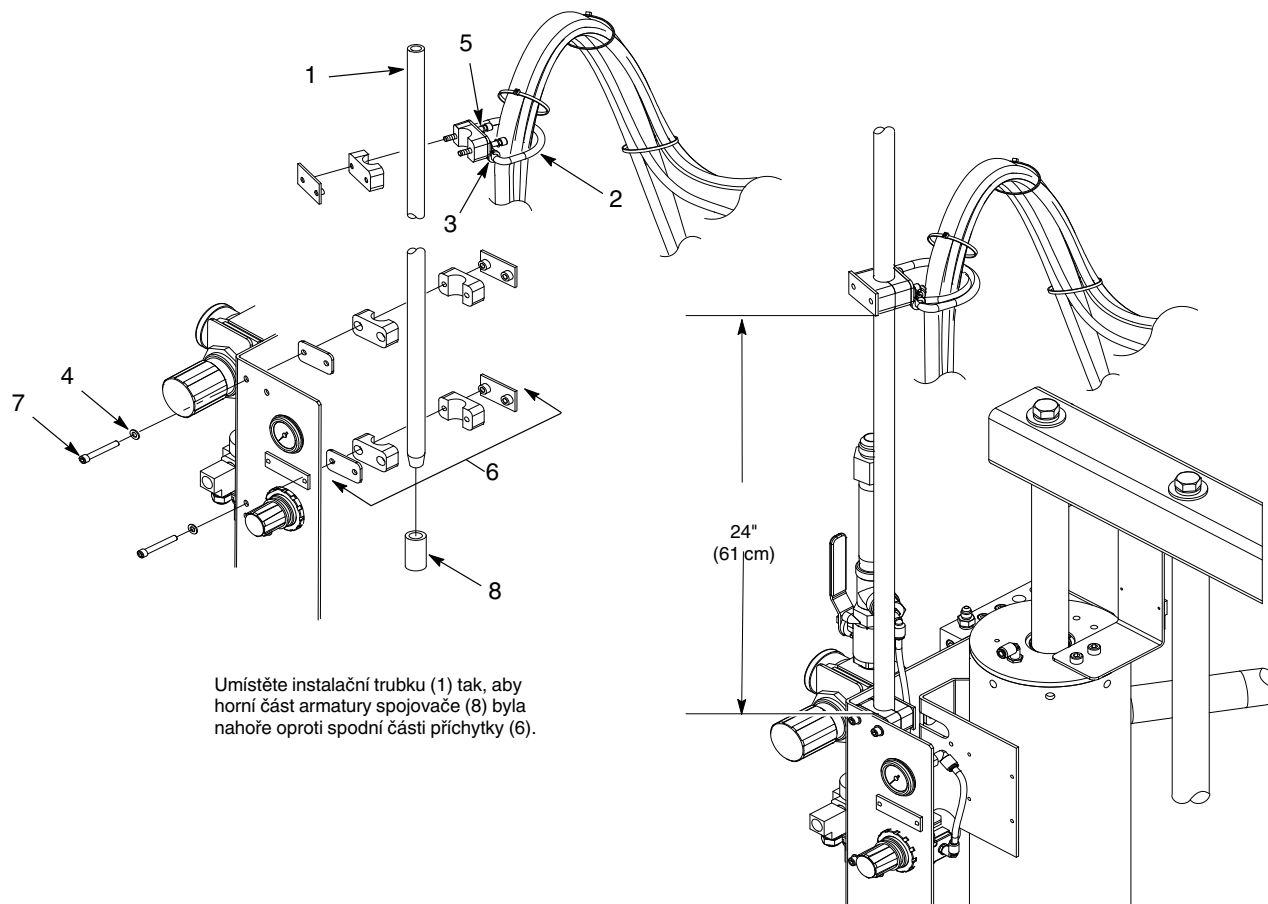
Obr. 1 Typické instalace Rhino SD2/XD2
