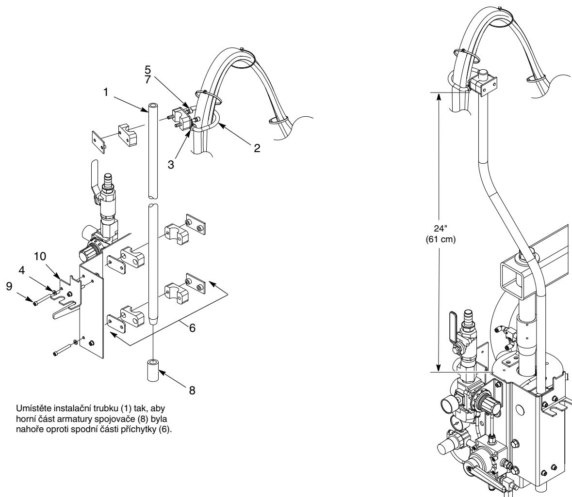
Obr. 2 Typické instalace podpory hadice Rhino VE
