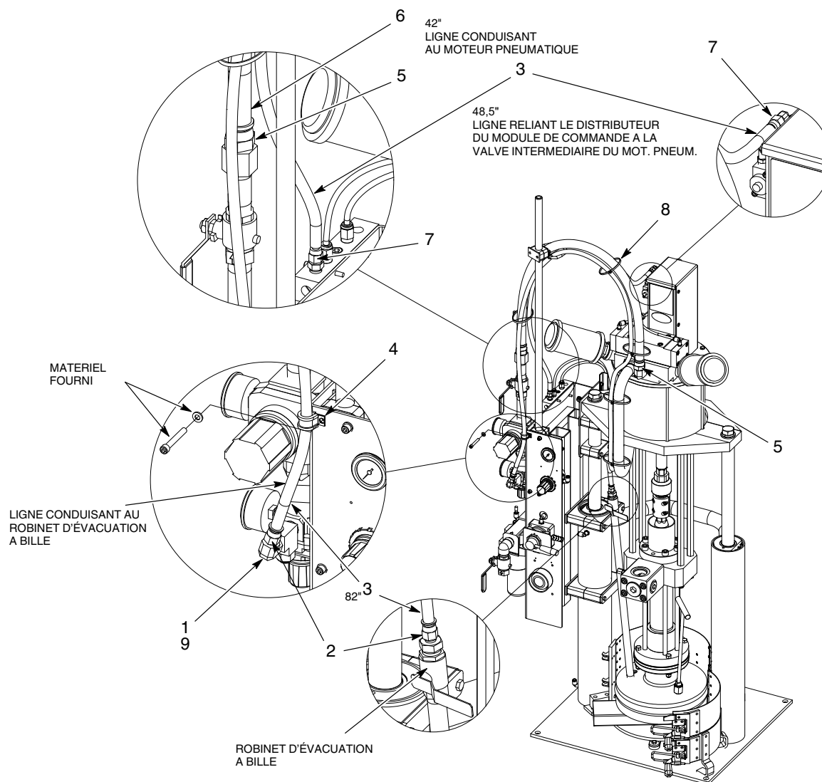
Figure 2 Module de tuyaux d'interconnexion ignifuges à petit châssis
