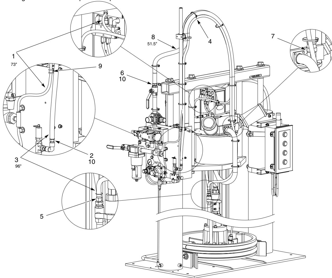
Figure 11 Grand châssis 55 gallons (210 l) Tuyau ignifuge vert
