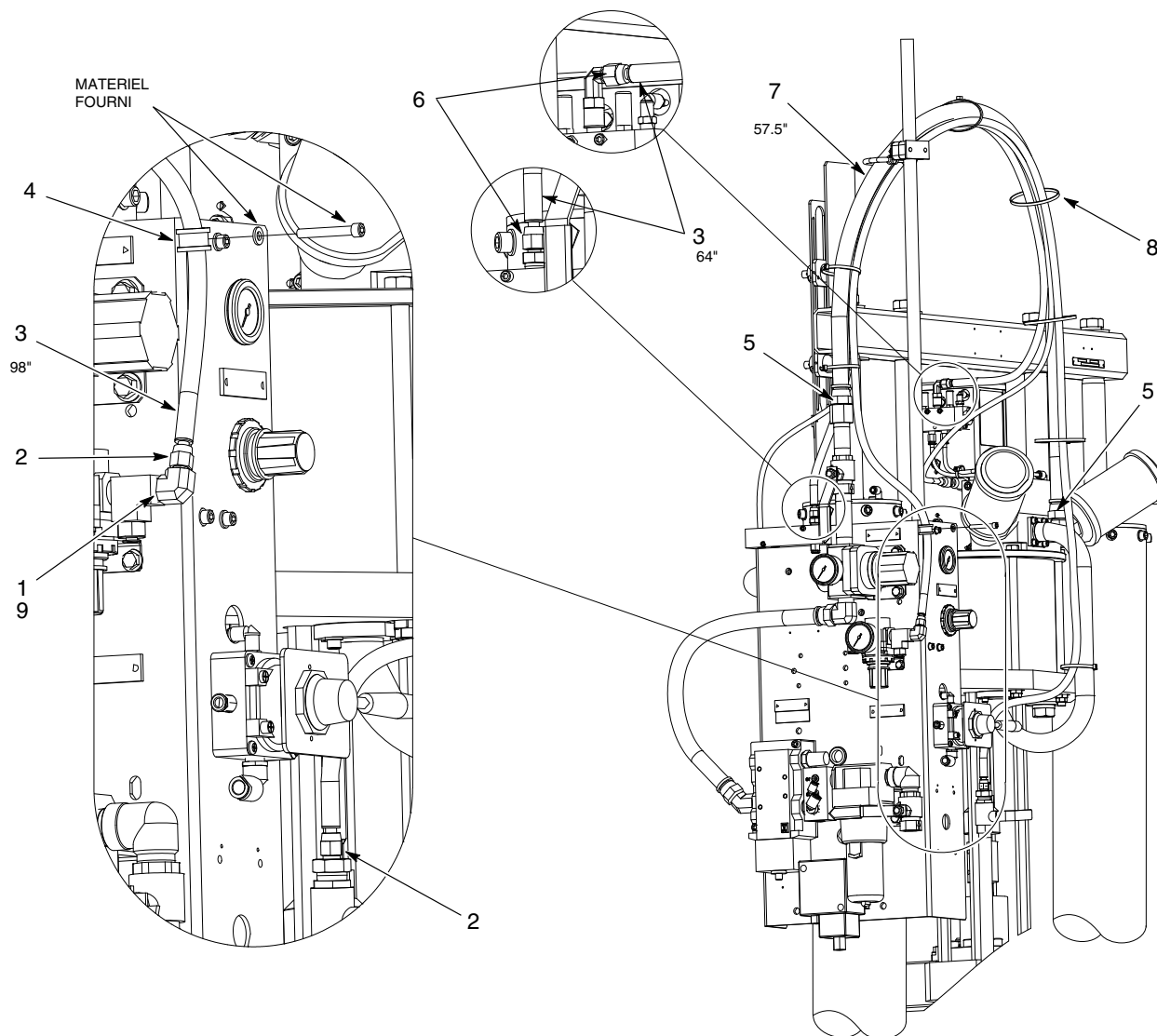
Figure 4 Tuyau ignifuge grand châssis 5/30 gallons (20/115 l)
