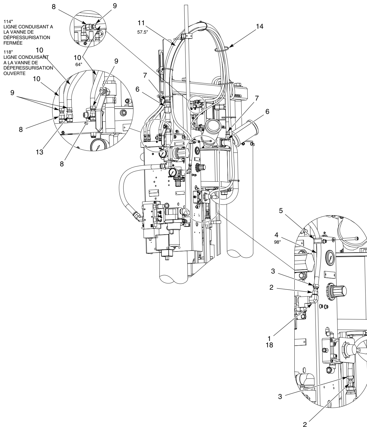
Figure 15 Grand châssis 55 gallons (210 l) Tuyau noir avec dépressurisation
