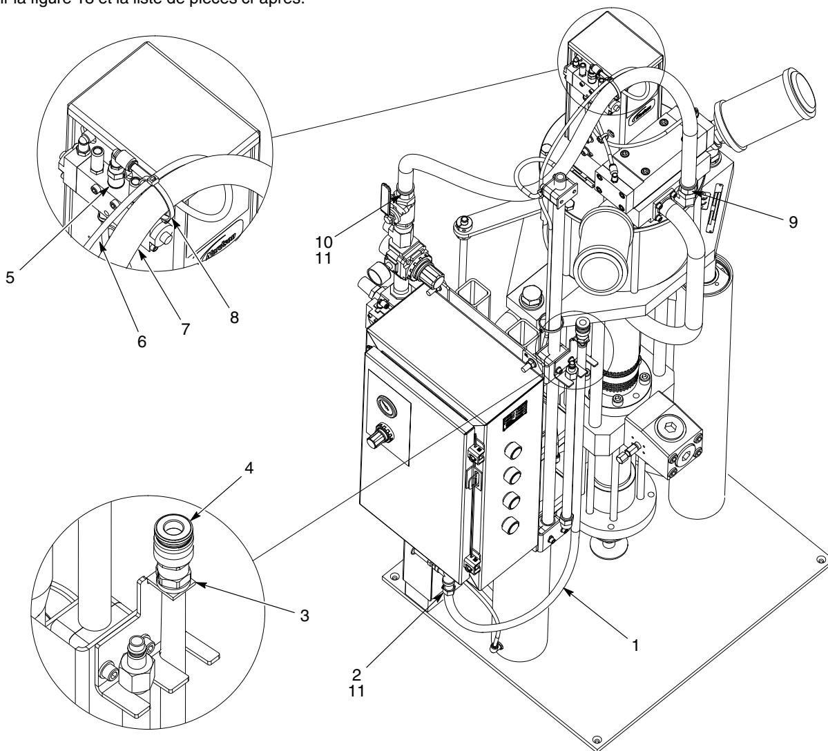
Figure 18 Tuyau CE petit châssis Rhino VE
