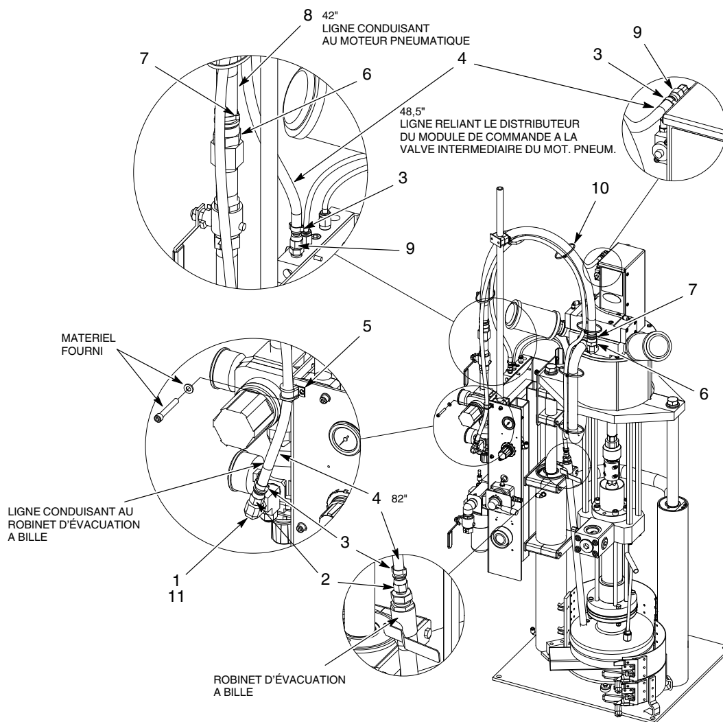
Figure 3 Tuyau noir pour petit châssis
