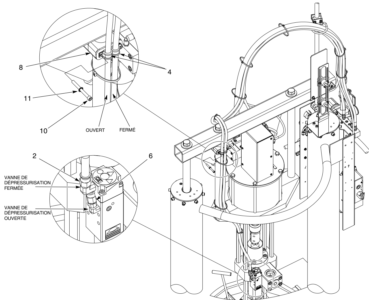
Figure 7 Tuyau ignifuge avec dépressurisation grand châssis 5/30 gallons (20/115 l) (suite)
