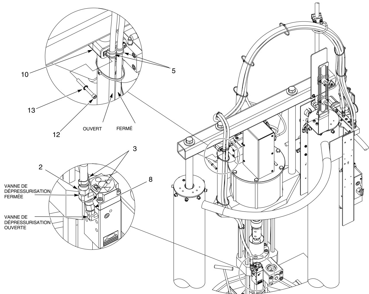
Figure 9 Tuyau noir avec dépressurisation grand châssis 5/30 gallons (20/115 l) (suite)
