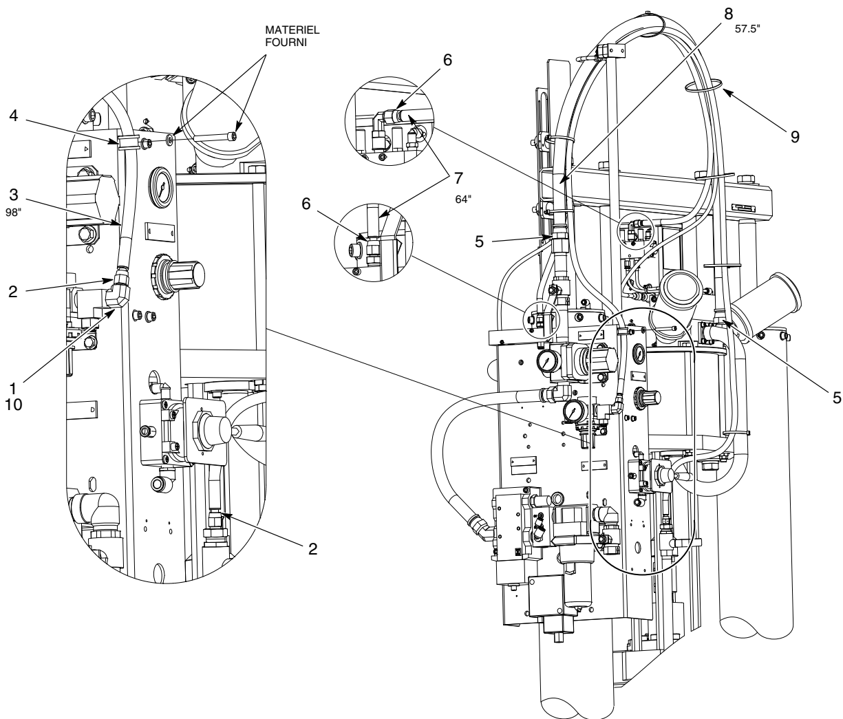
Figure 10 Tuyau ignifuge grand châssis 55 gallons (210 l)
