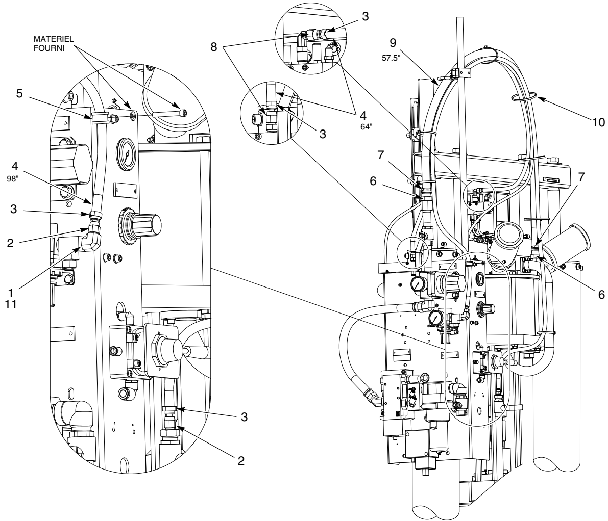
Figure 5 Tuyau ignifuge grand châssis 5/30 gallons (20/115 l)
