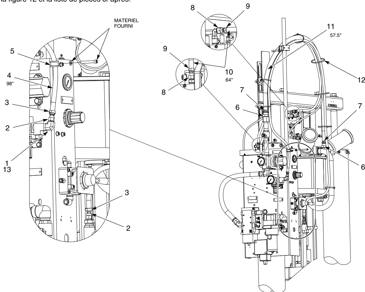
Figure 12 Tuyau noir grand châssis 55 gallons (210 l)
