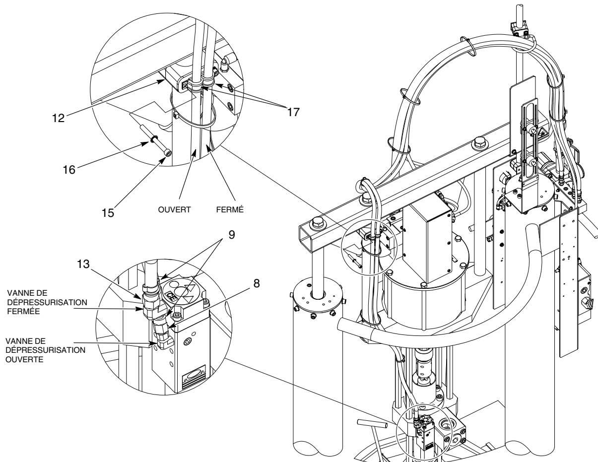
Figure 16 Tuyau noir avec dépressurisation grand châssis 55 gallons (210 l) (suite)
