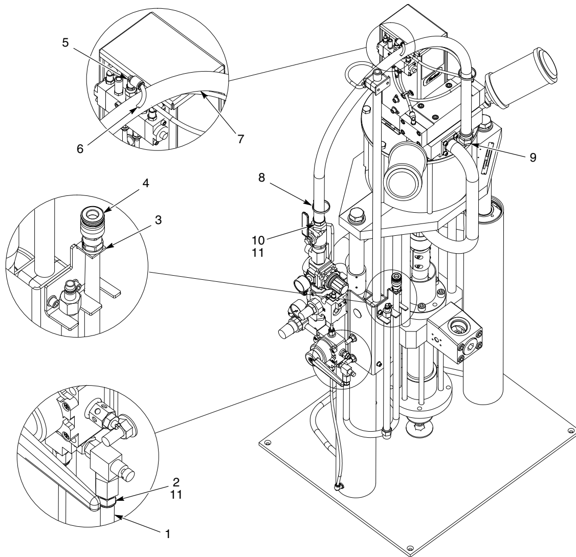
Figure 17 Tuyau petit châssis Rhino VE
