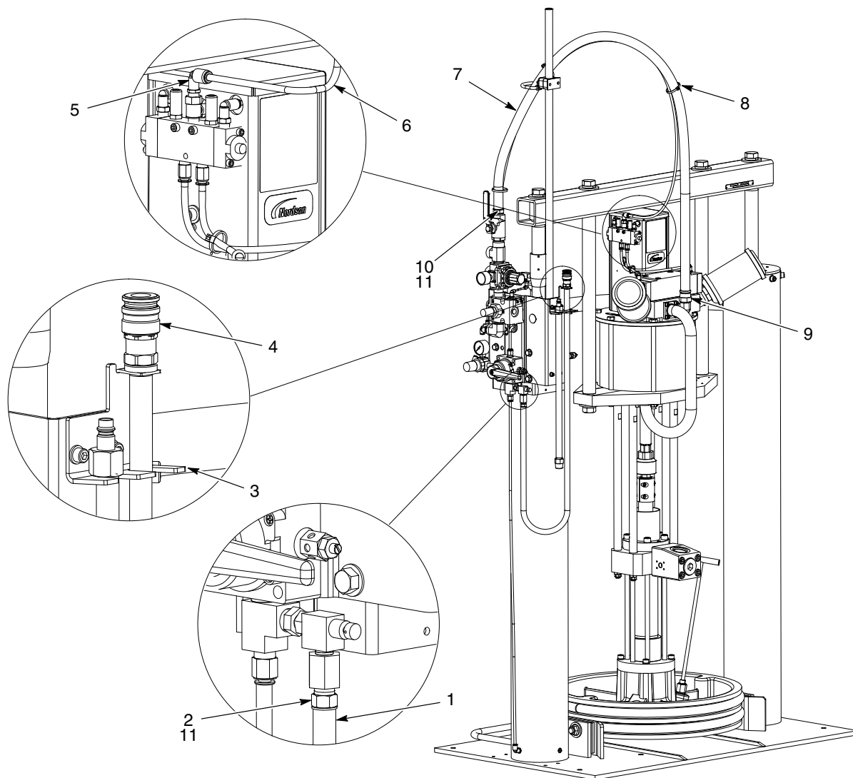
Rys. 19 Wąż do dużej ramy do urządzenia Rhino VE
