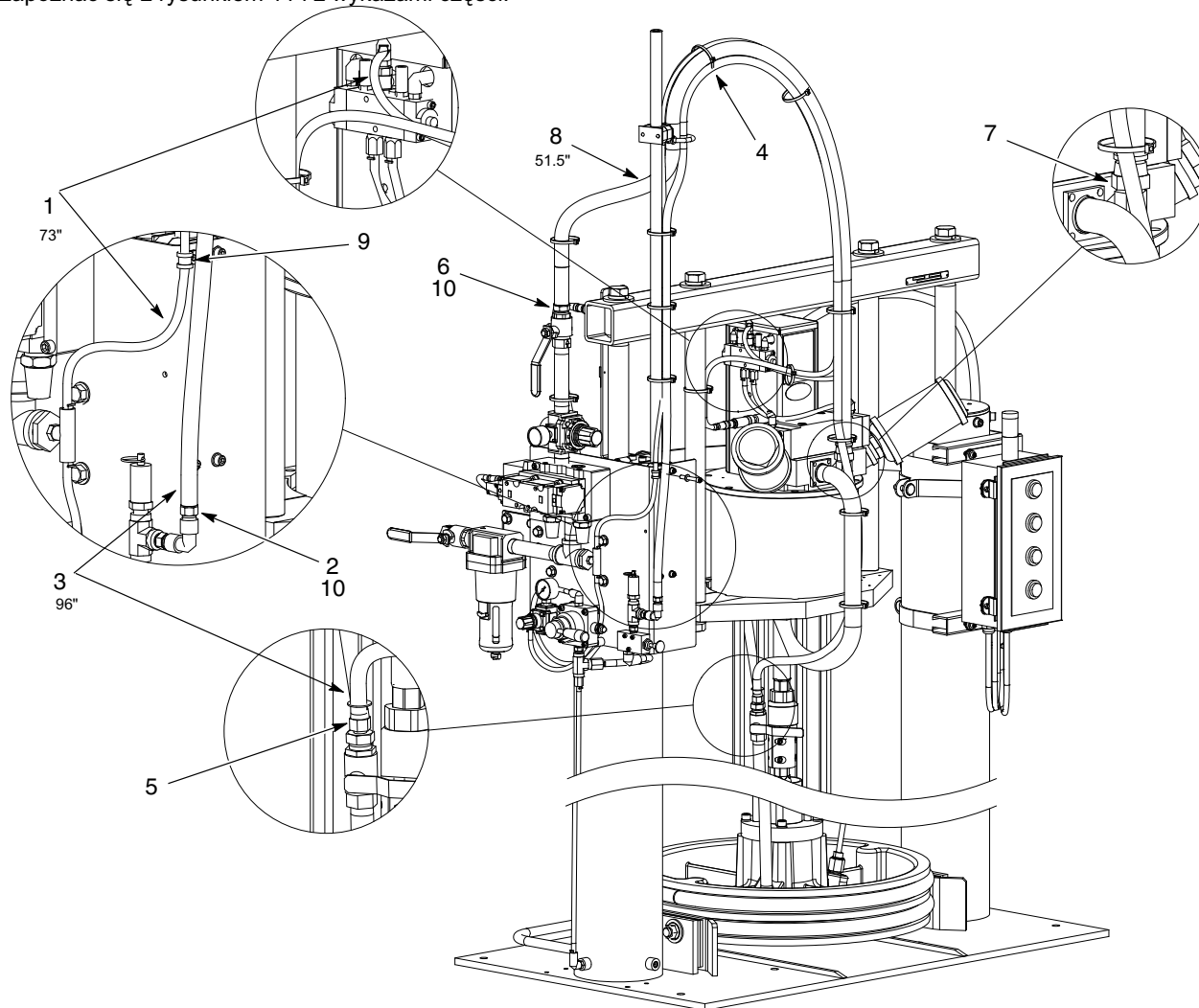
Rys. 11 Zielony węży ogniotrwały do dużej ramy do beczek o pojemności 55 galonów
