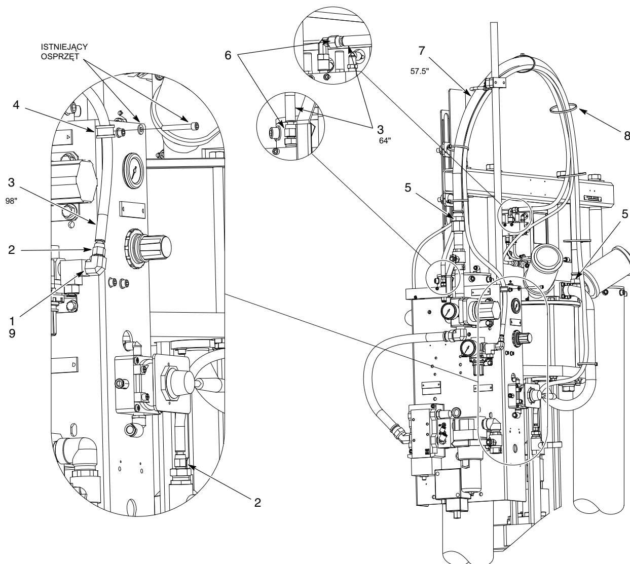
Rys. 4 Wąż ogniotrwały do dużej ramy do beczek o pojemności 5/30 galonów
