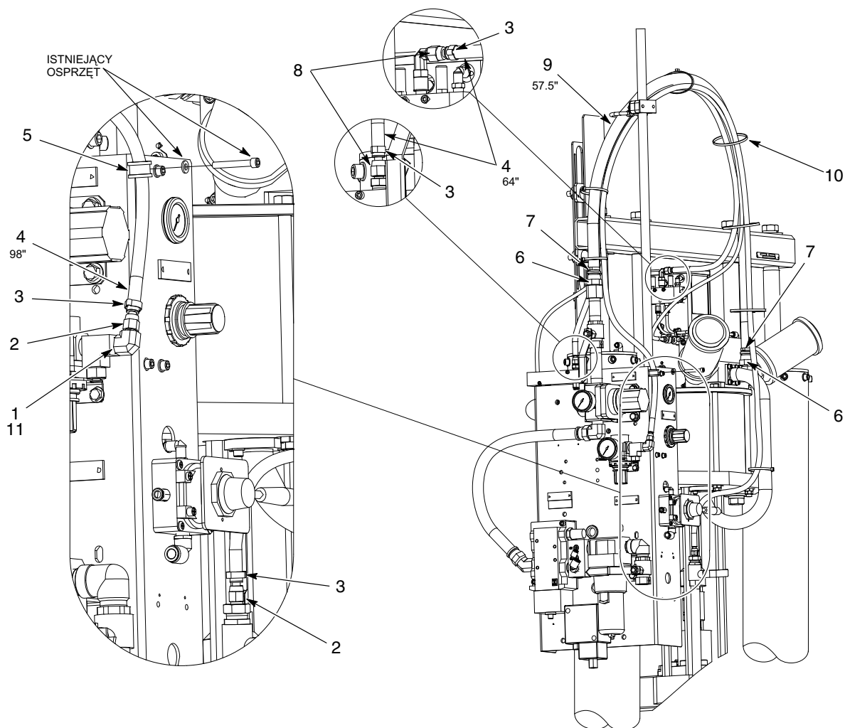
Rys. 5 Czarny wąż do dużej ramy do beczek o pojemności 5/30 galonów
