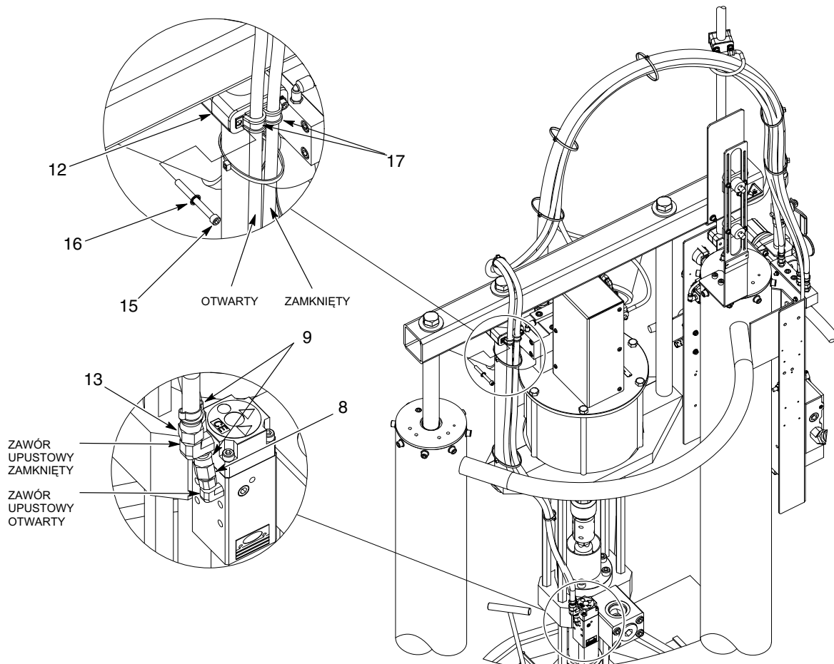
Rys. 16 Czarny wąż do dużej ramy do beczek o pojemności 55 galonów z możliwością odpuszczenia ciśnienia (cd.)
