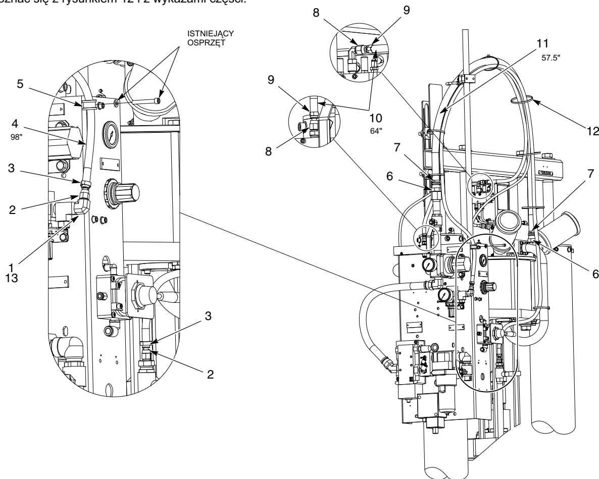
Rys. 12 Czarny wąż do dużej ramy do beczek o pojemności 55 galonów
