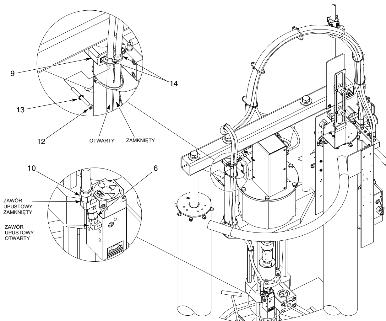
Rys. 14 Czarny węży do dużej ramy do beczek o pojemności 55 galonów (cd.)
