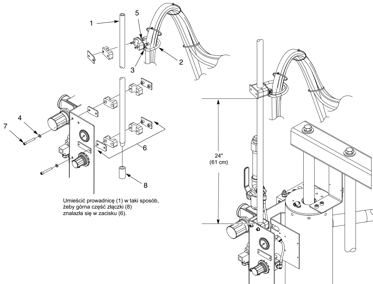
Rys. 1 Typowa instalacja Rhino SD2/XD2
