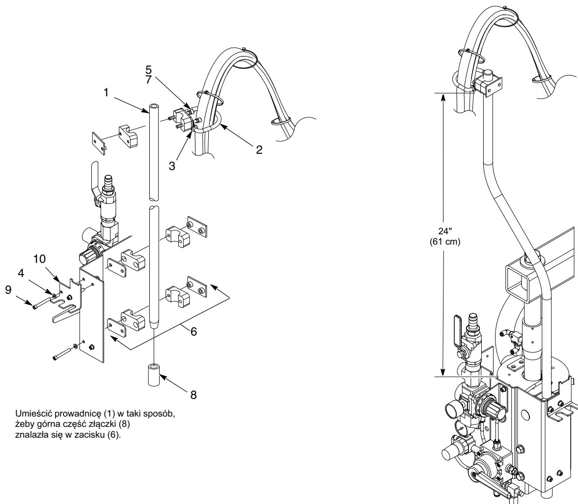
Rys. 2 Typowa instalacja modułu wspornika węża VE
