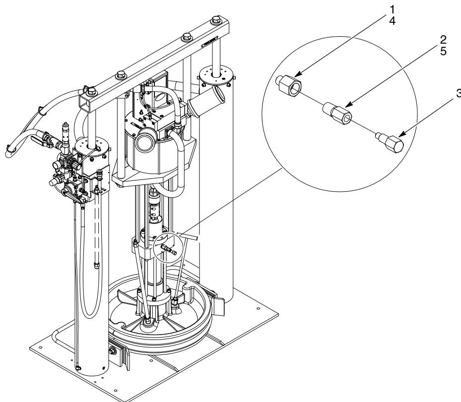
Rysunek 1 Zawór upustowy Rhino VE
