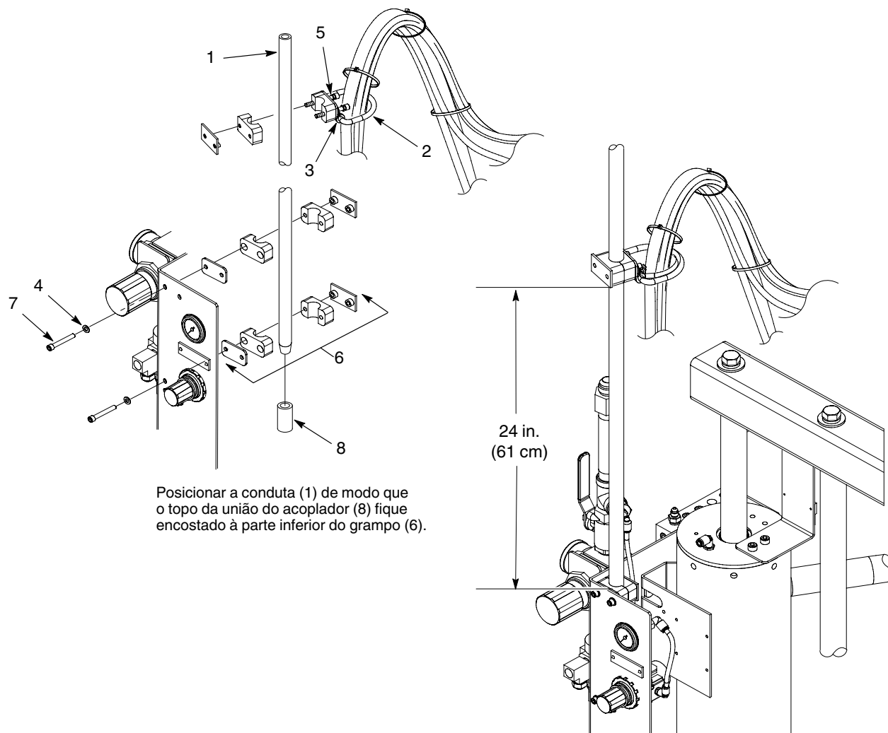
Figura 1 Instalação típica
