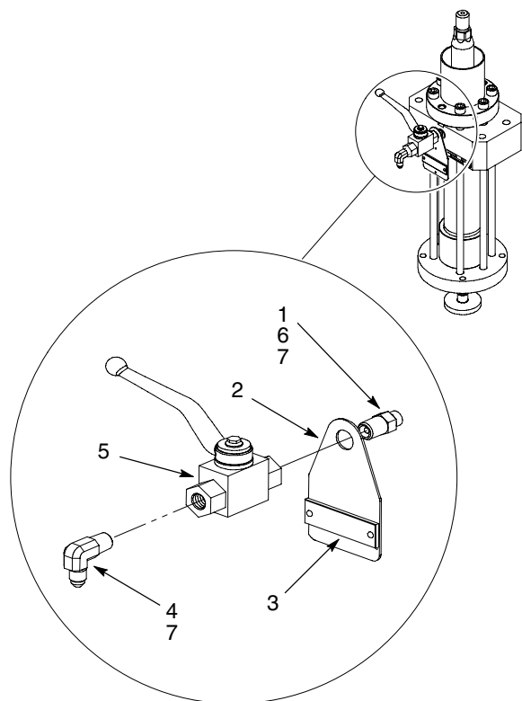
Figura 4 Válvula de purga para soporte de 30/55 galones
