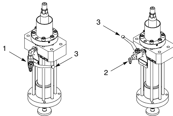
Figura 1 Válvulas de purga de bola típicas
