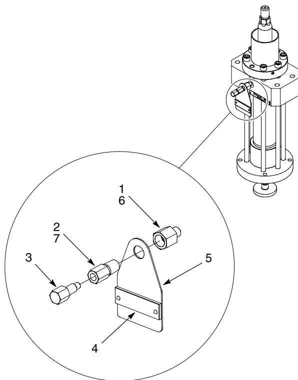
Figura 5 Válvula de purga
