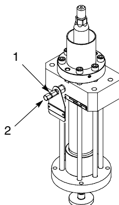
Figura 2 Válvulas de purga de aguja y asiento
