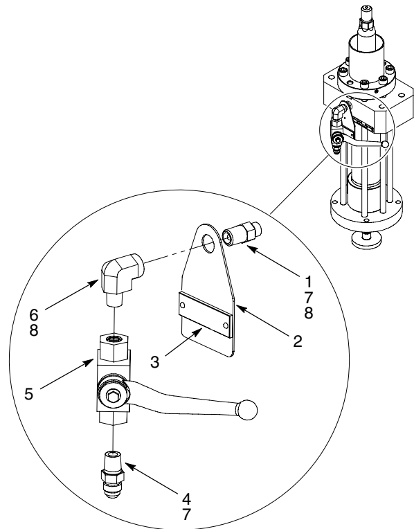
Figura 3 Válvula de purga para soporte de cubo de 5 galones
