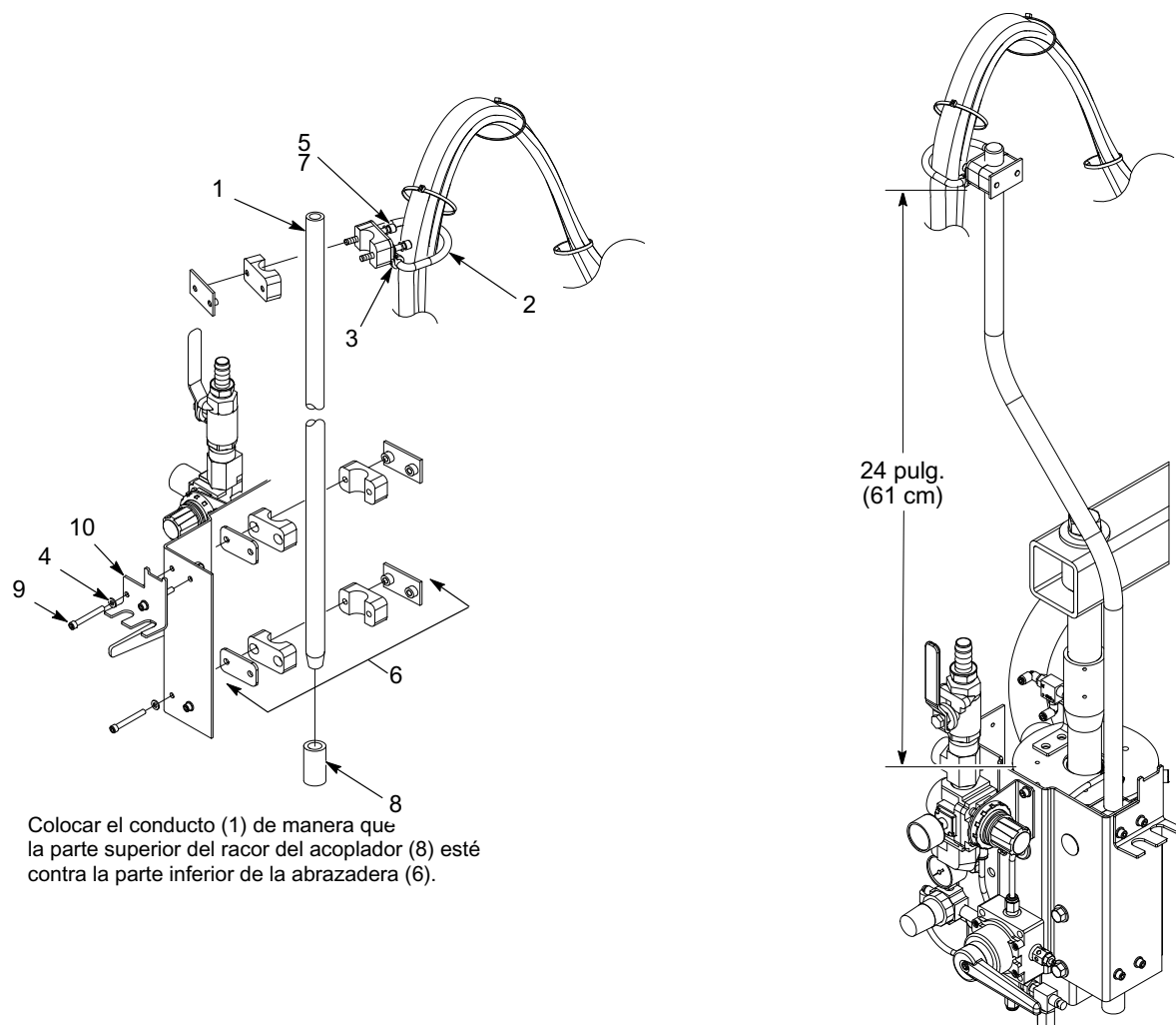
Figura 2 Instalación típica de soporte de manguera VE de Rhino
