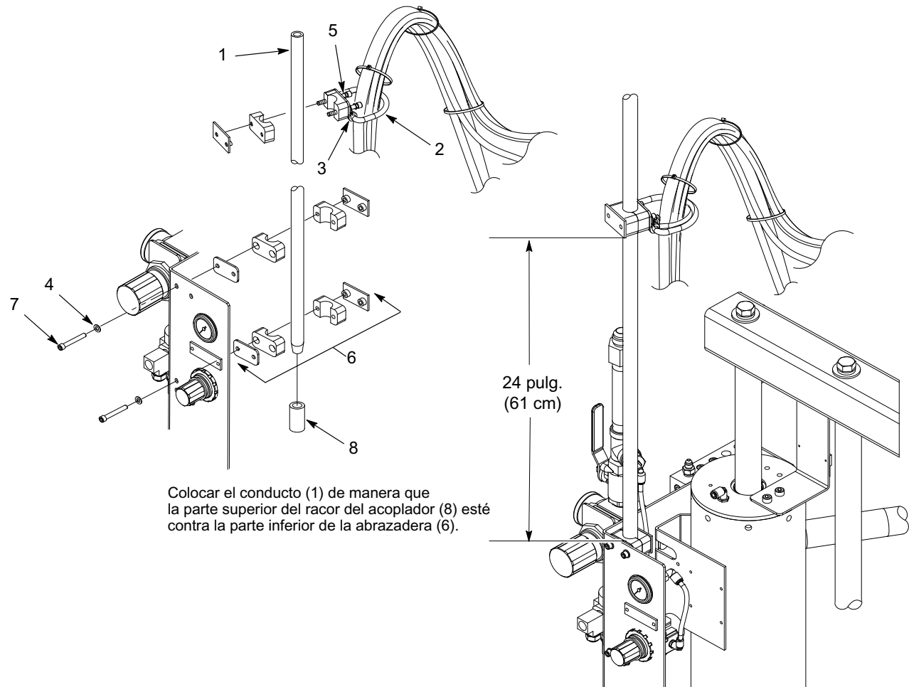
Figura 1 Instalación típica SD2/XD2 de Rhino
