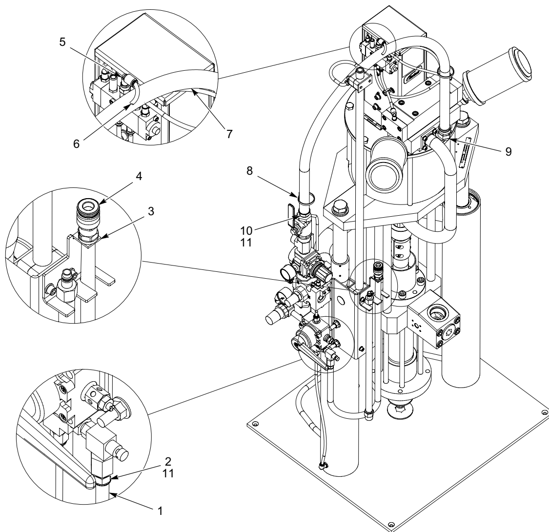
Figura 17 Manguera para soporte pequeño VE de Rhino
