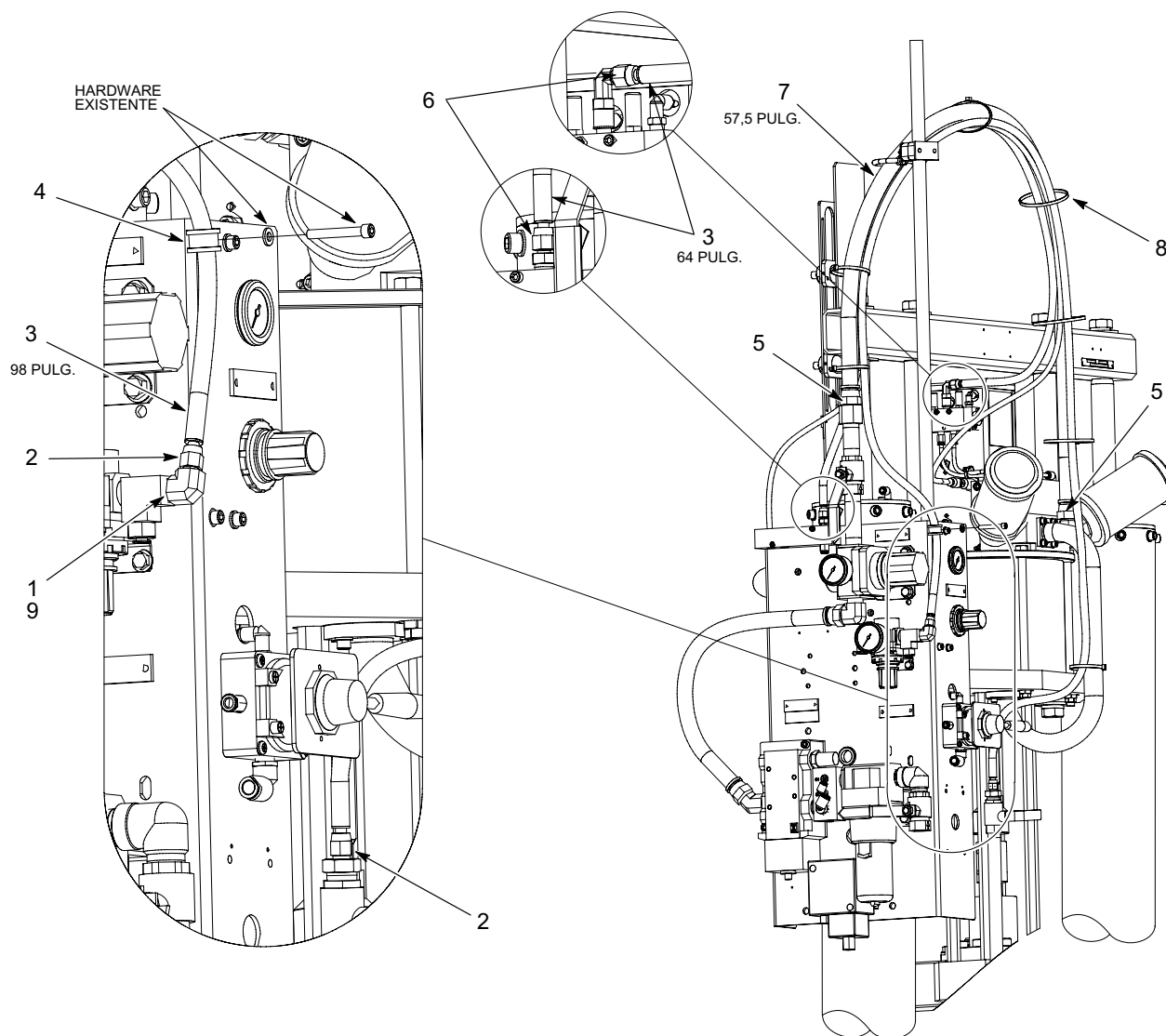
Figura 4 Manguera resistente al fuego para soporte grande de 5/30 galones
