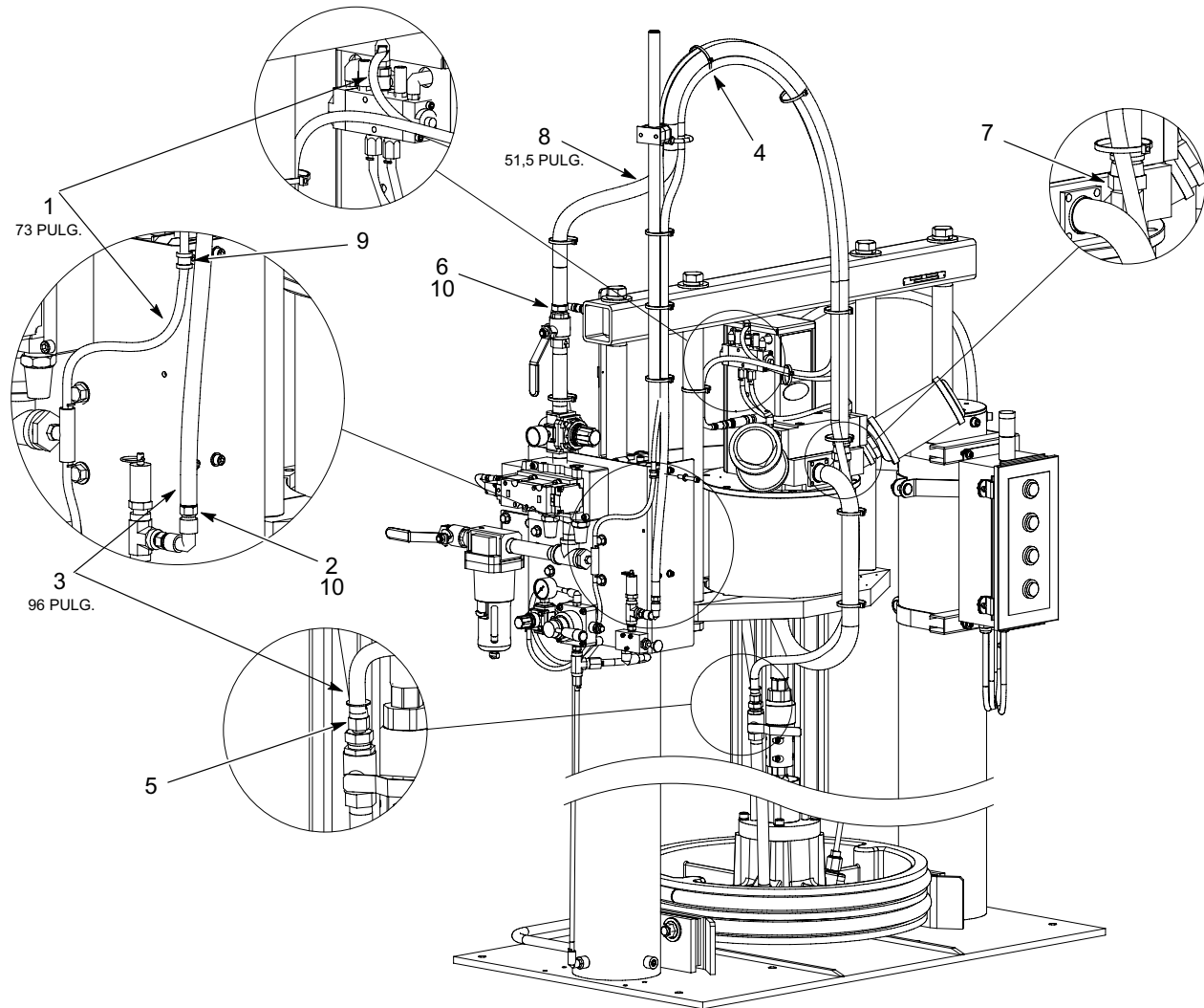
Figura 11 Manguera verde resistente al fuego para soporte grande de 55 galones
