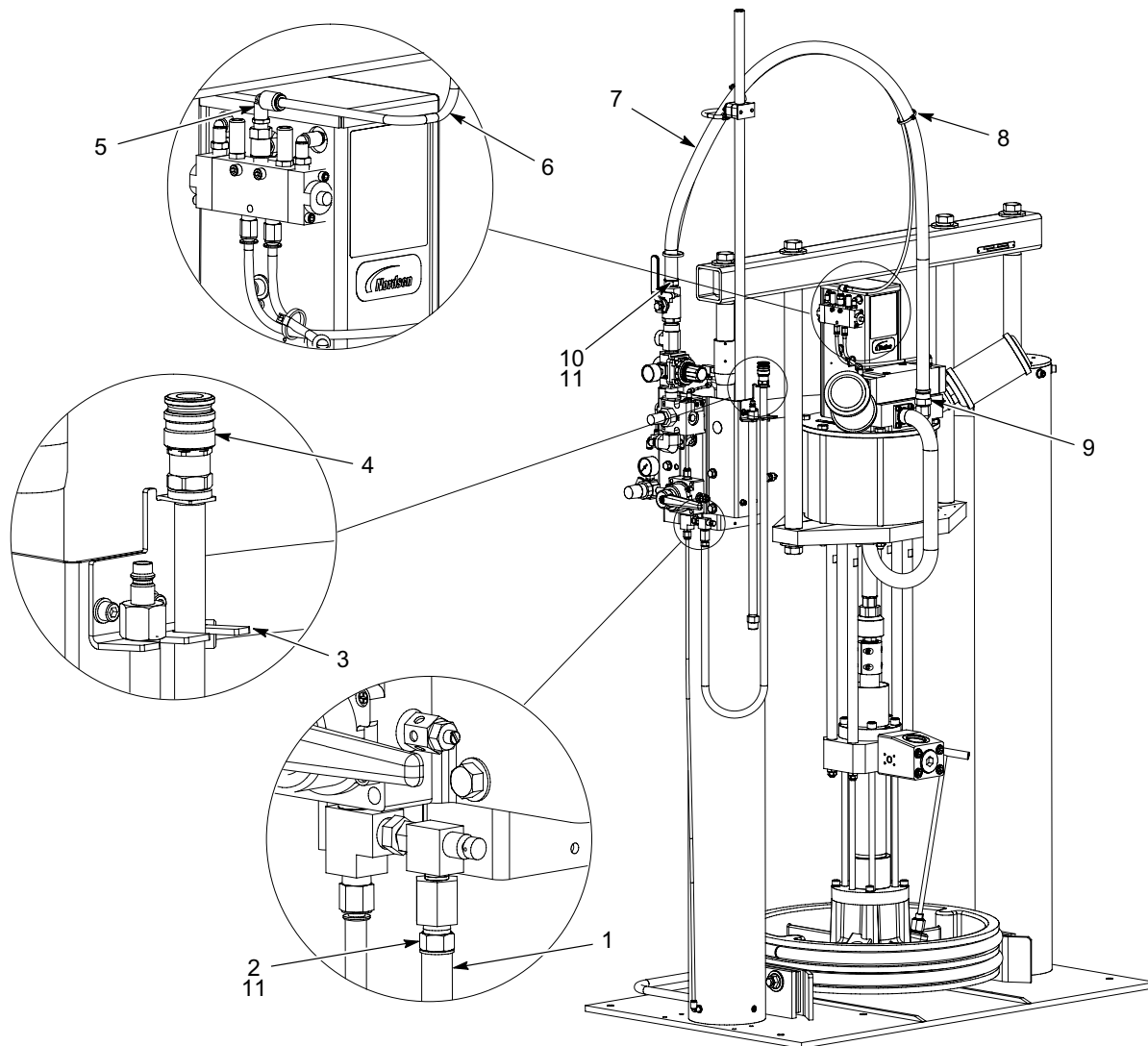
Figura 19 Manguera CE para soporte grande VE de Rhino
