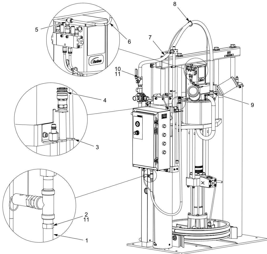
Figura 20 Manguera CE para soporte grande VE de Rhino
