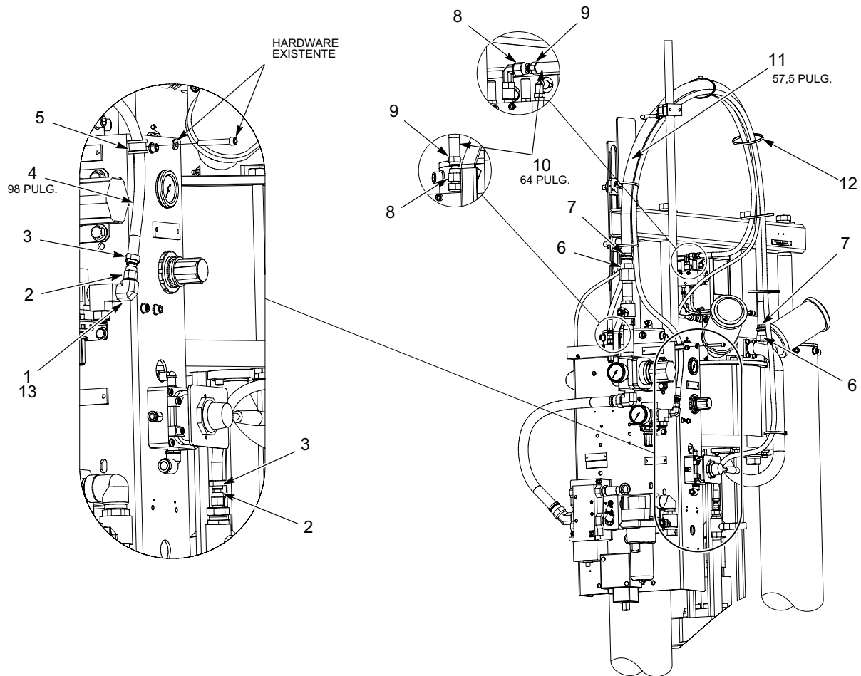
Figura 12 Manguera negra para soporte grande de 55 galones
