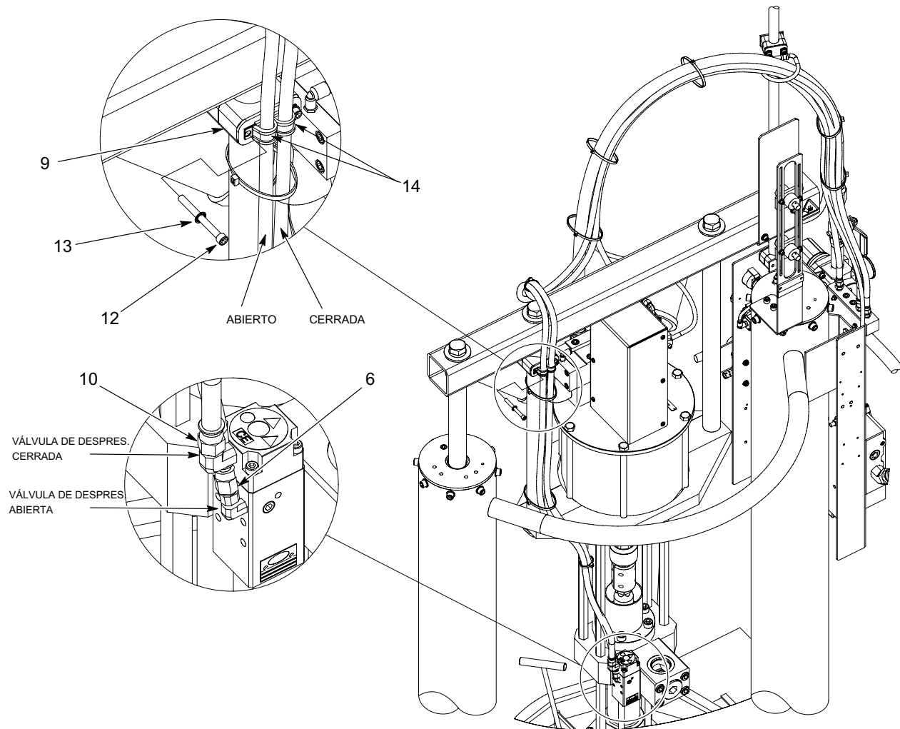
Figura 14 Manguera negra para soporte grande de 55 galones (continuación)
