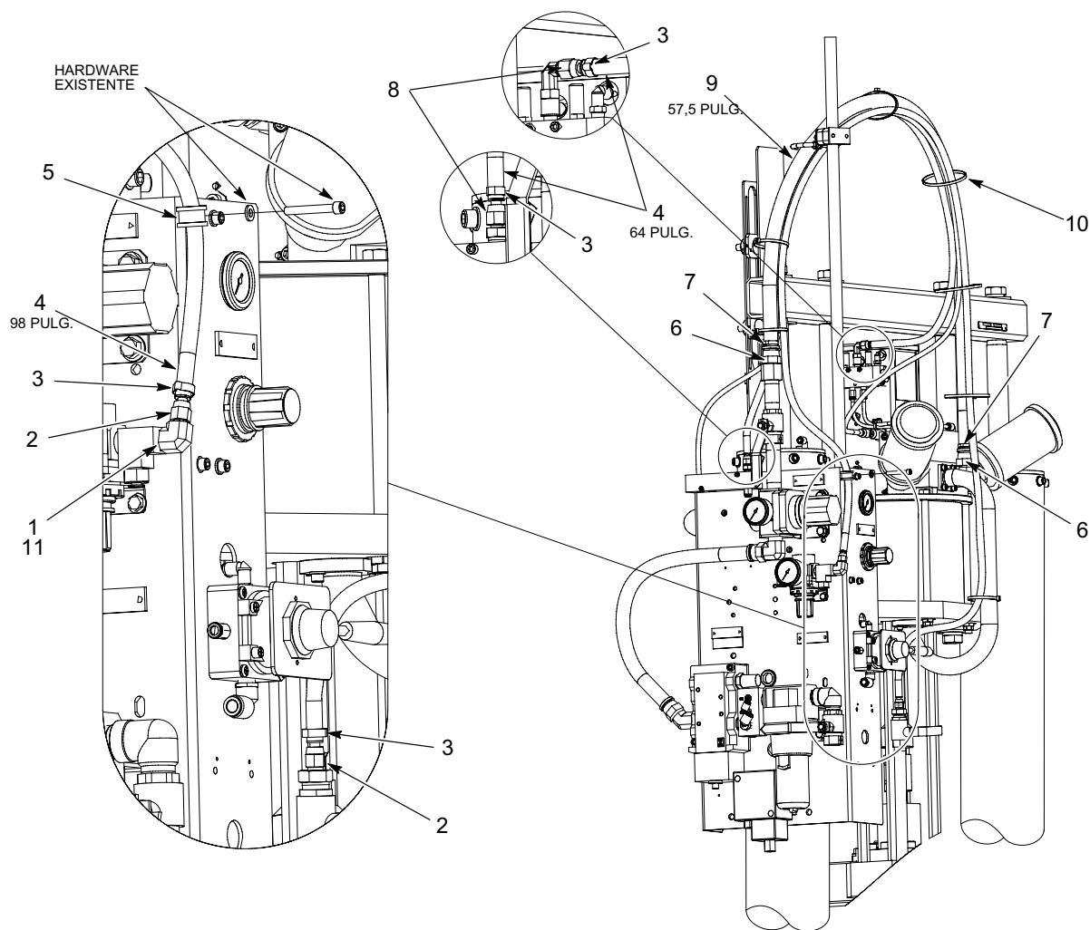
Figura 5 Manguera negra para soporte grande de 5/30 galones
