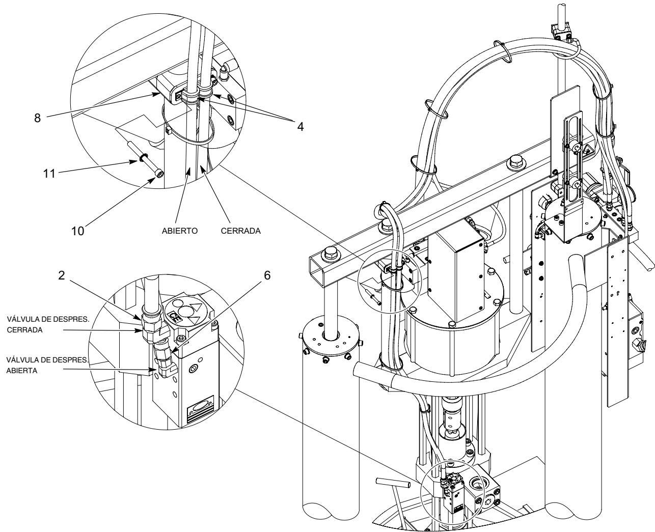
Figura 7 Manguera resistente al fuego para soporte grande de 5/30 galones con despresurización (continuación)
