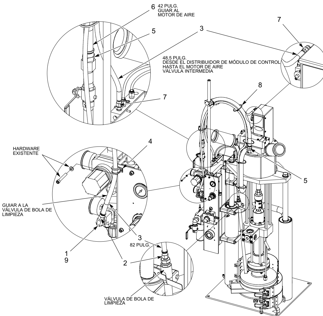
Figura 2 Módulo de manguera de interconexión resistente al fuego para soporte pequeño
