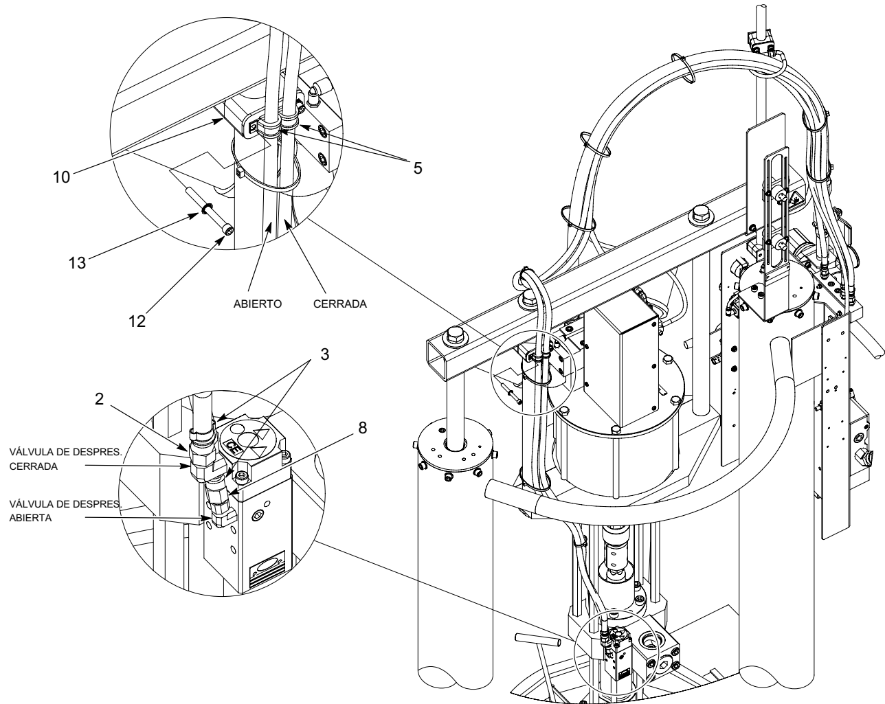
Figura 9 Manguera negra para soporte grande de 5/30 galones con despresurización (continuación)
