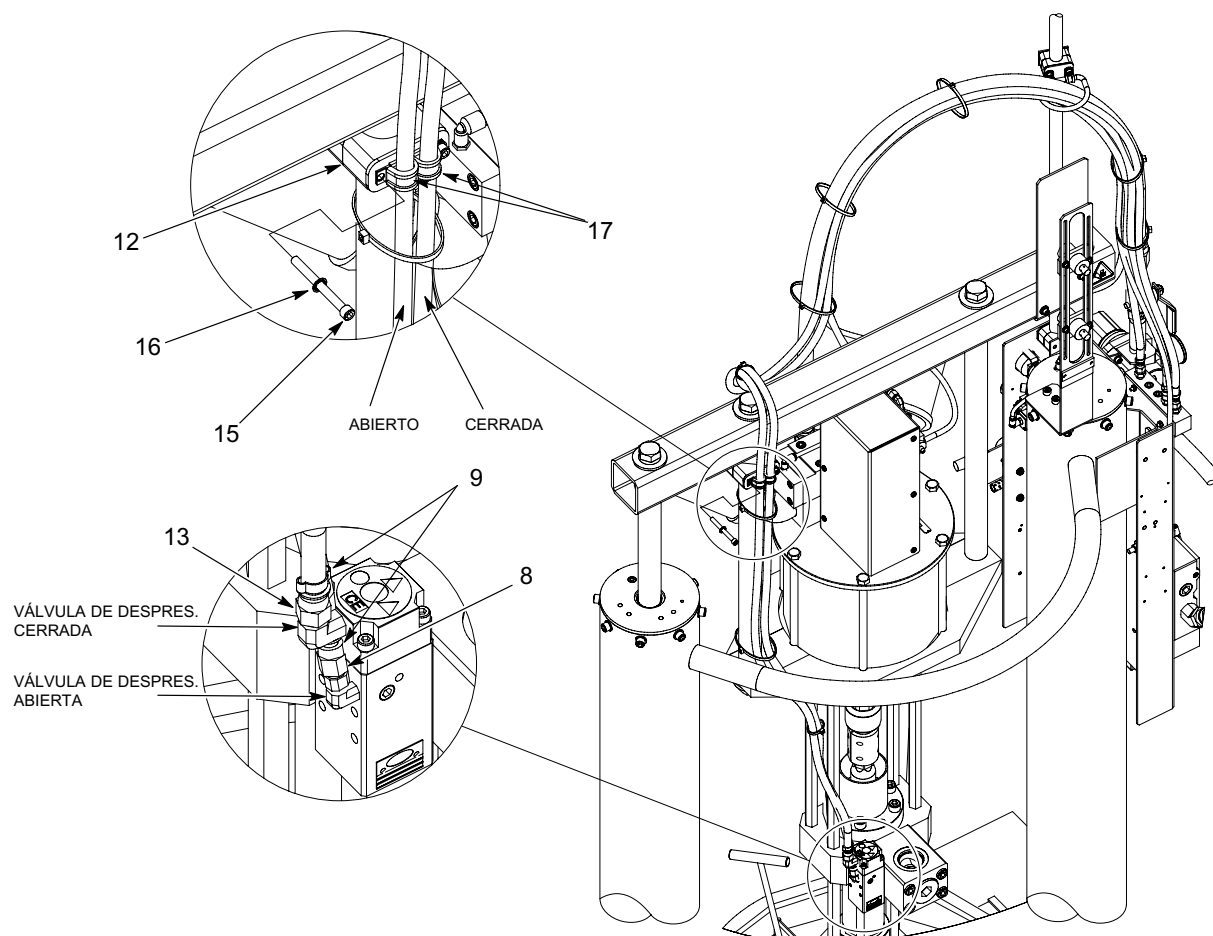
Figura 16 Manguera negra para soporte grande de 55 galones con despresurización (continuación)
