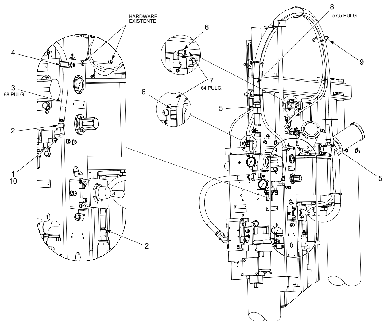
Figura 10 Manguera resistente al fuego para soporte grande de 55 galones
