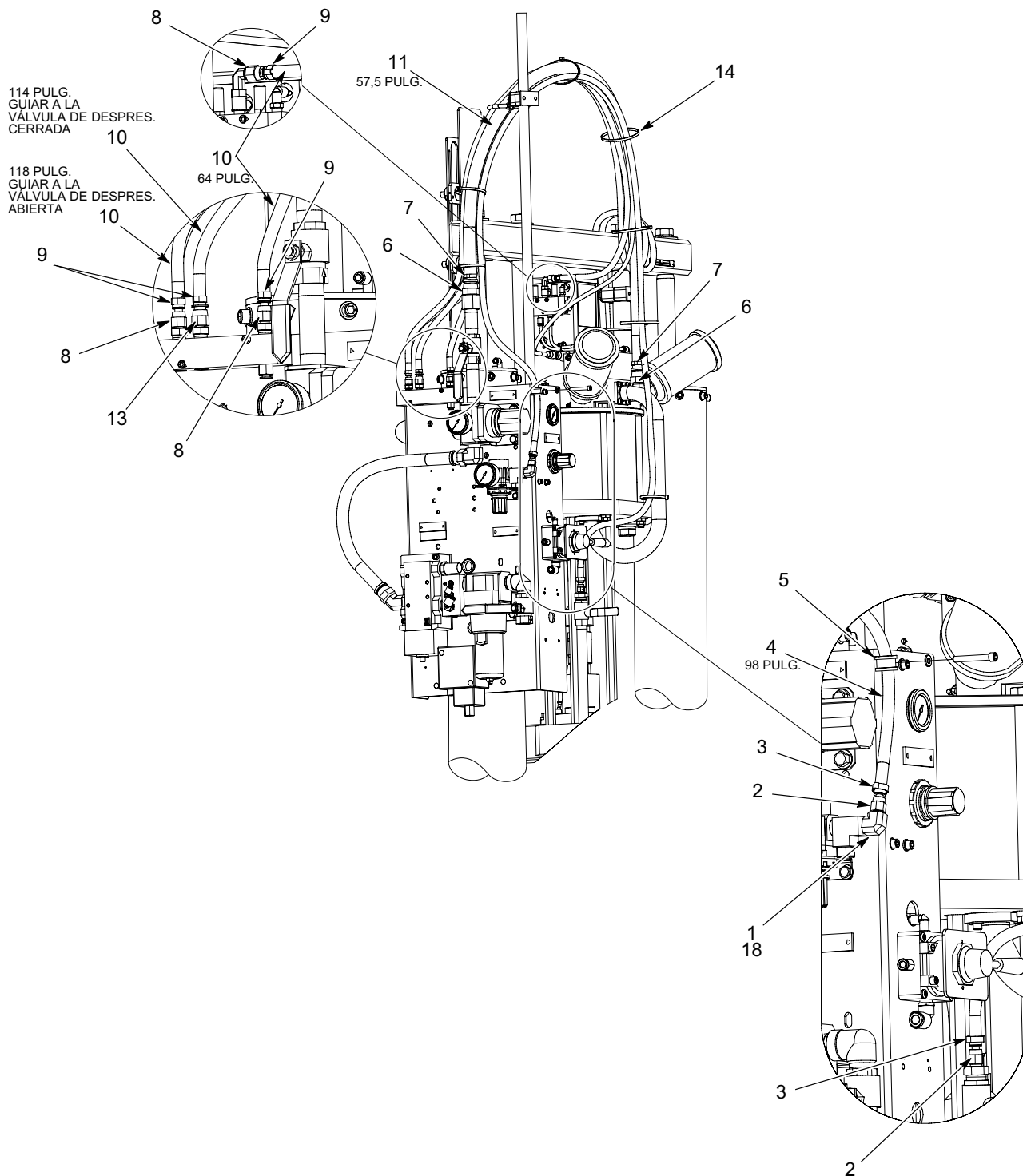
Figura 15 Manguera negra para soporte grande de 55 galones con despresurización
