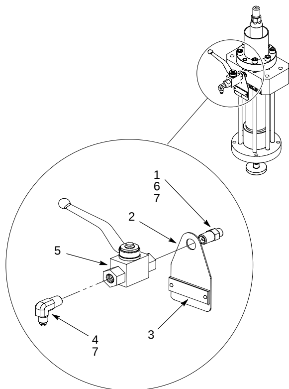
Figura 4 Supape de aerisire a cadrului de 30/55 galoane
