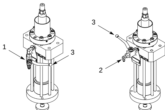
Figura 1 Supape de aerisire cu bilă obișnuite
