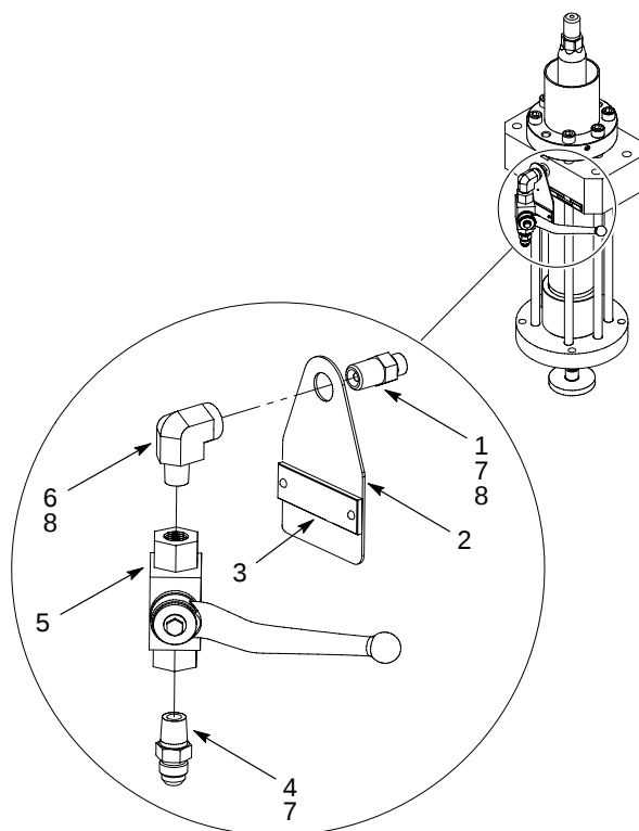
Figura 3 Supapă de aerisire a cadrului cupei de 5 galoane
