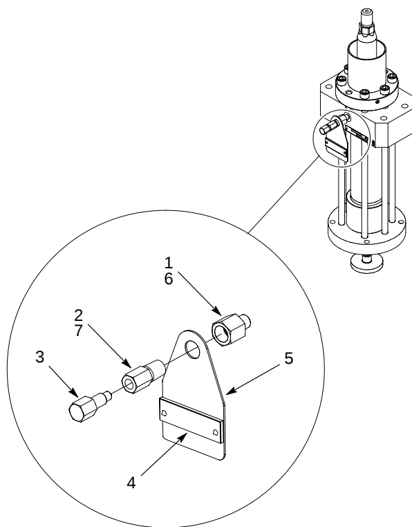
Figura 5 Supapă de aerisire
