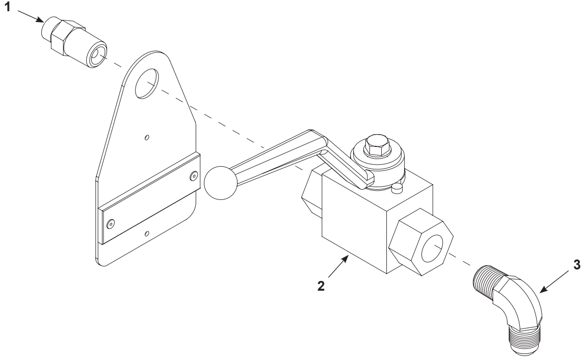
Şekil 5 Küresel valf, ön
