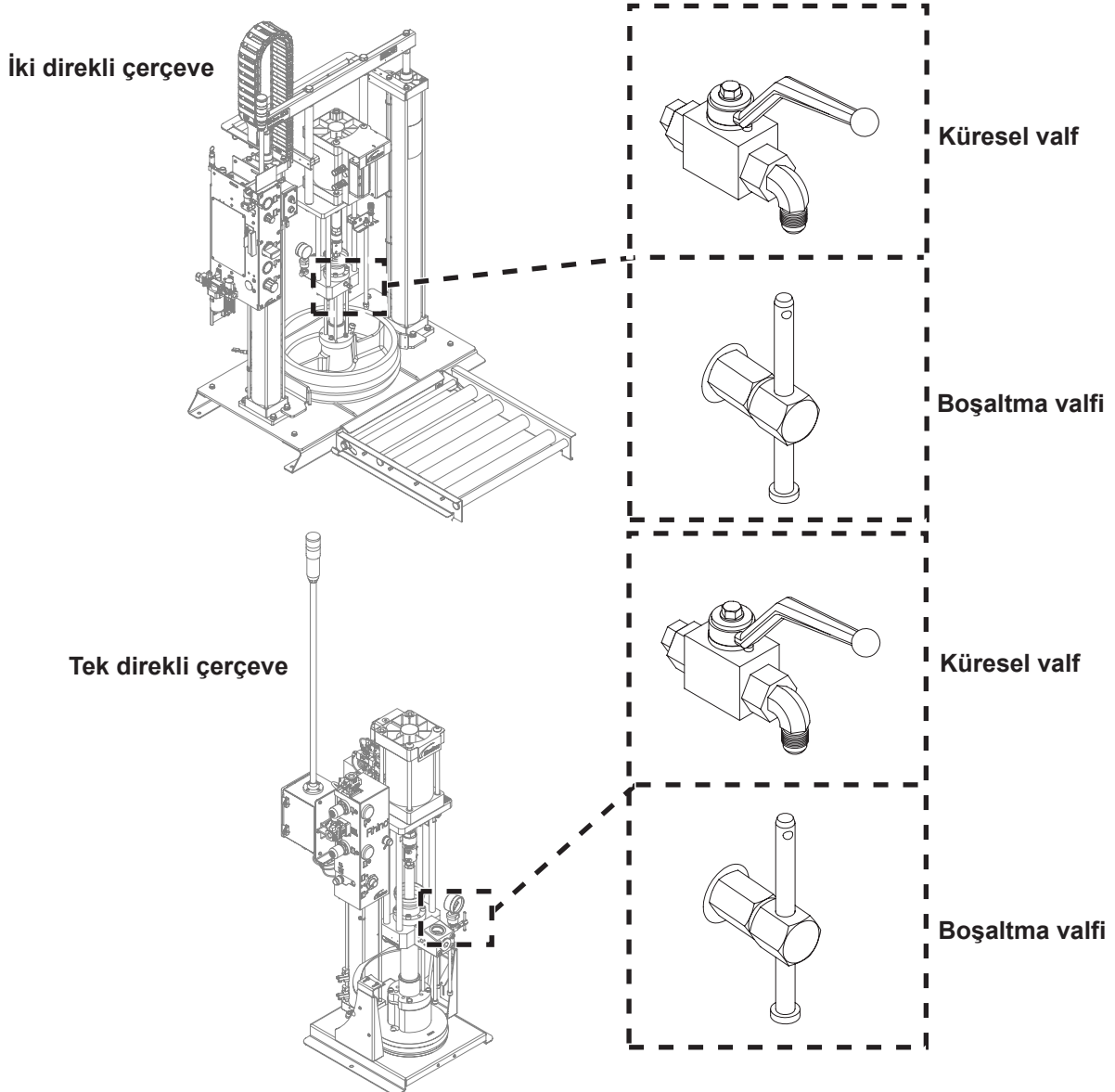
Şekil 1 Boşaltma valfinin/küresel valfin konumu
