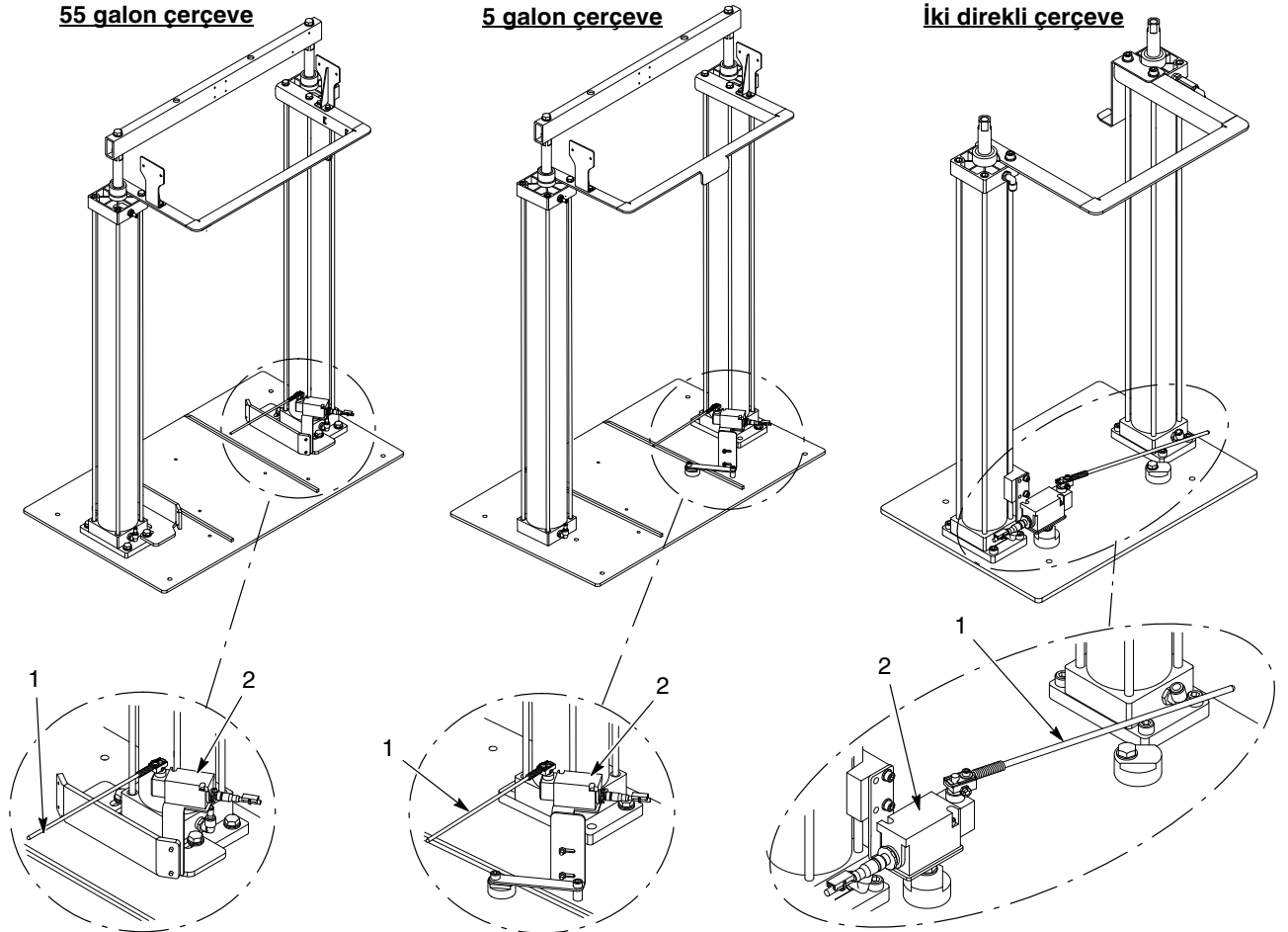
Şekil 1 Konteyner yerinde sensörü
