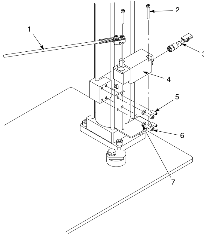
Şekil 5 İkili direk çerçeve konteyner yerinde sensörü
