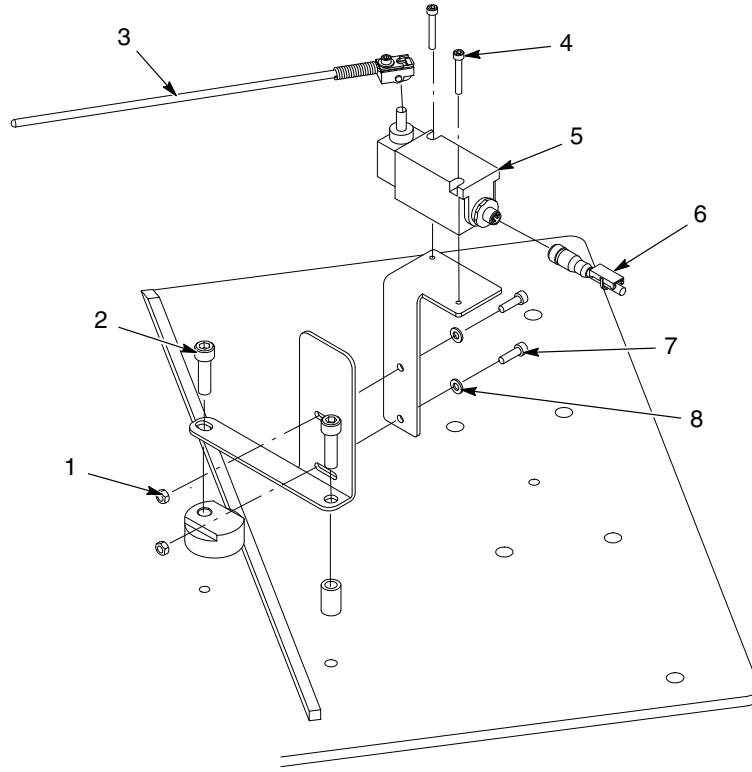
Şekil 4 5-galon çerçeve konteyner yerinde sensörü
