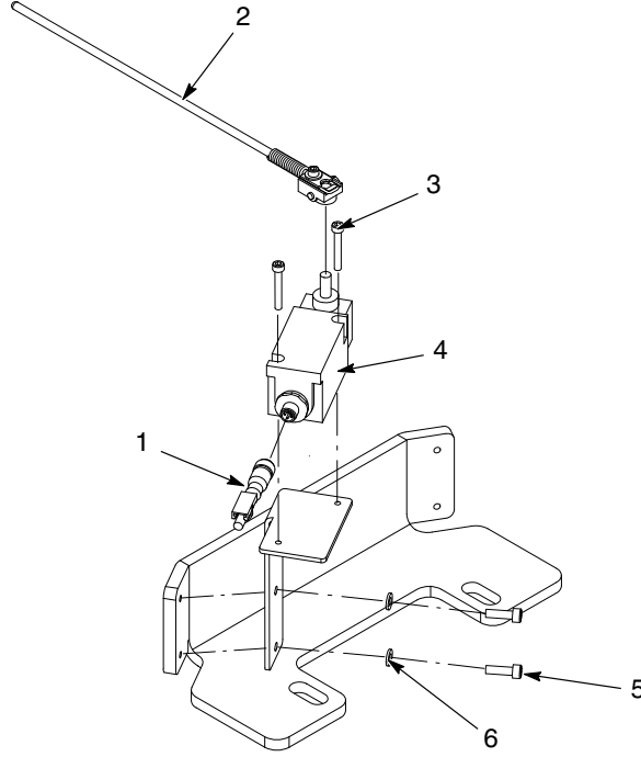
Şekil 3 55-galon çerçeve konteyner yerinde sensörü
