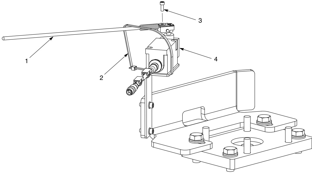
Şekil 2 Limit şalterinin ayarlanması
