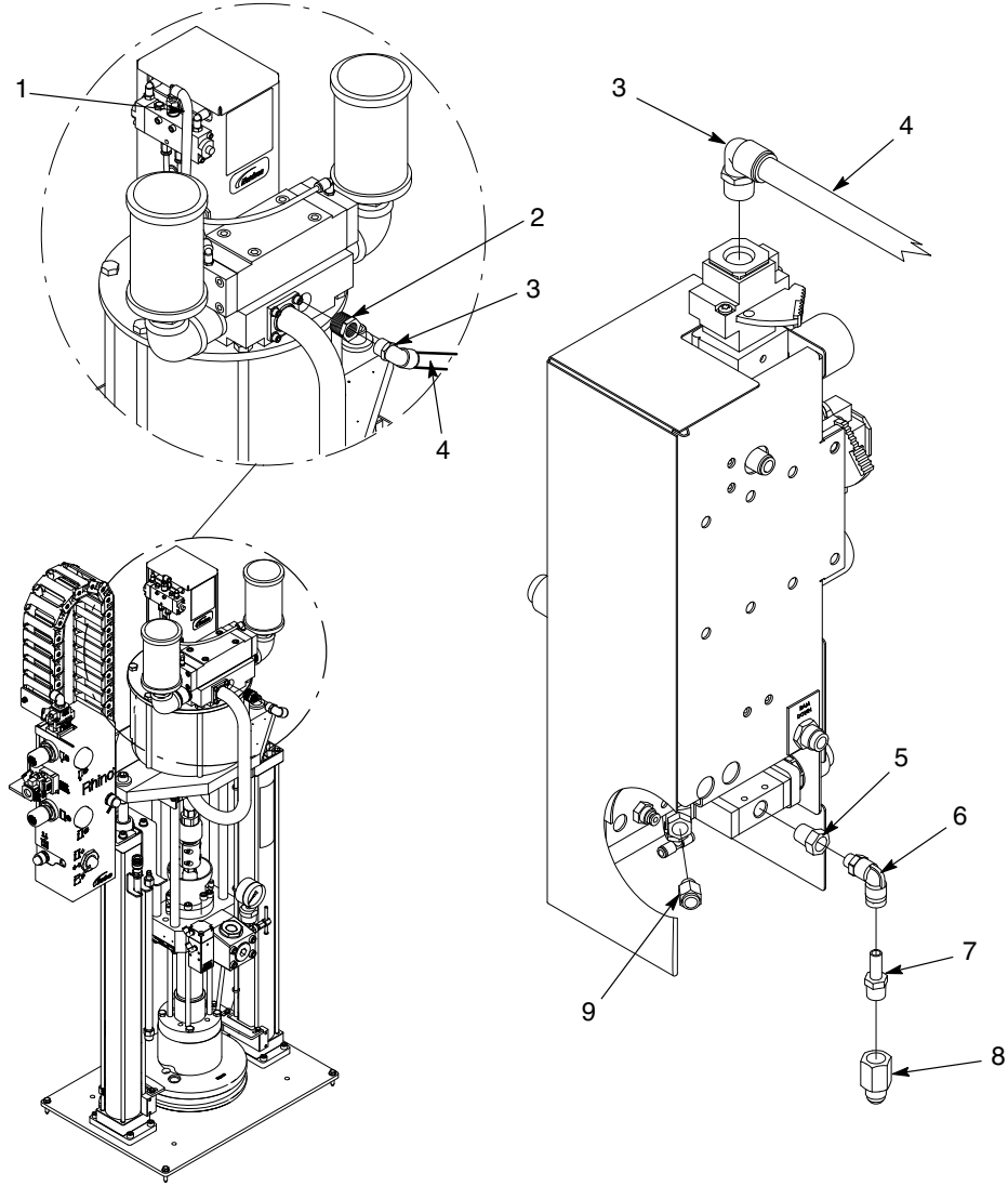
Şekil 21 SD2 hava motorlu DP çerçeve hortum modülü, pnömatik (2/2)
