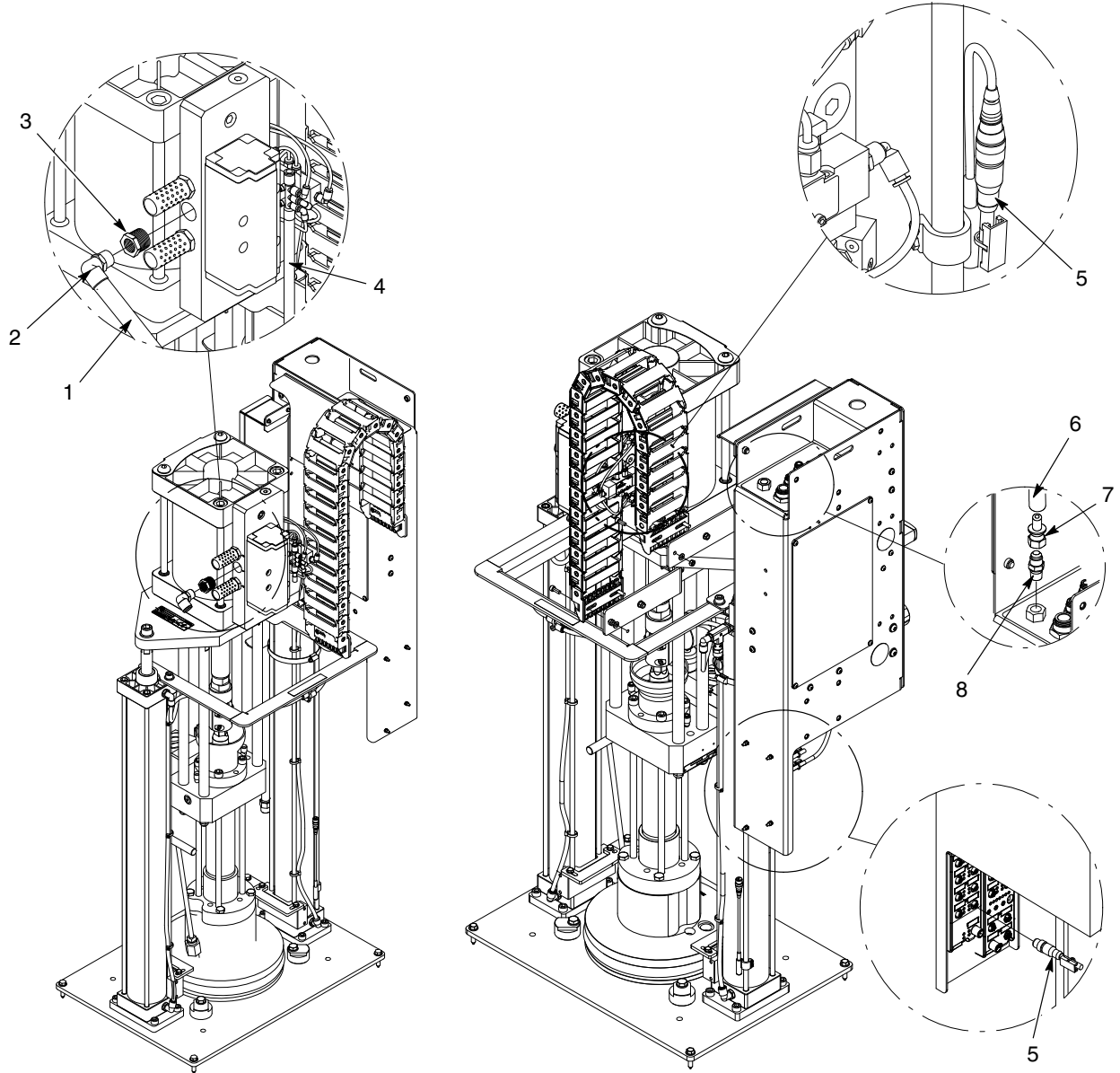
Şekil 4 SD3 hava motorlu DP çerçeve hortum modülü, 24 Vdc (1/2)
