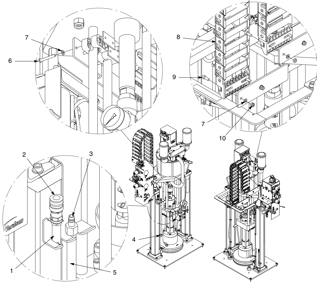
Şekil 20 SD2 hava motorlu DP çerçeve hortum modülü, pnömatik (1/2)
