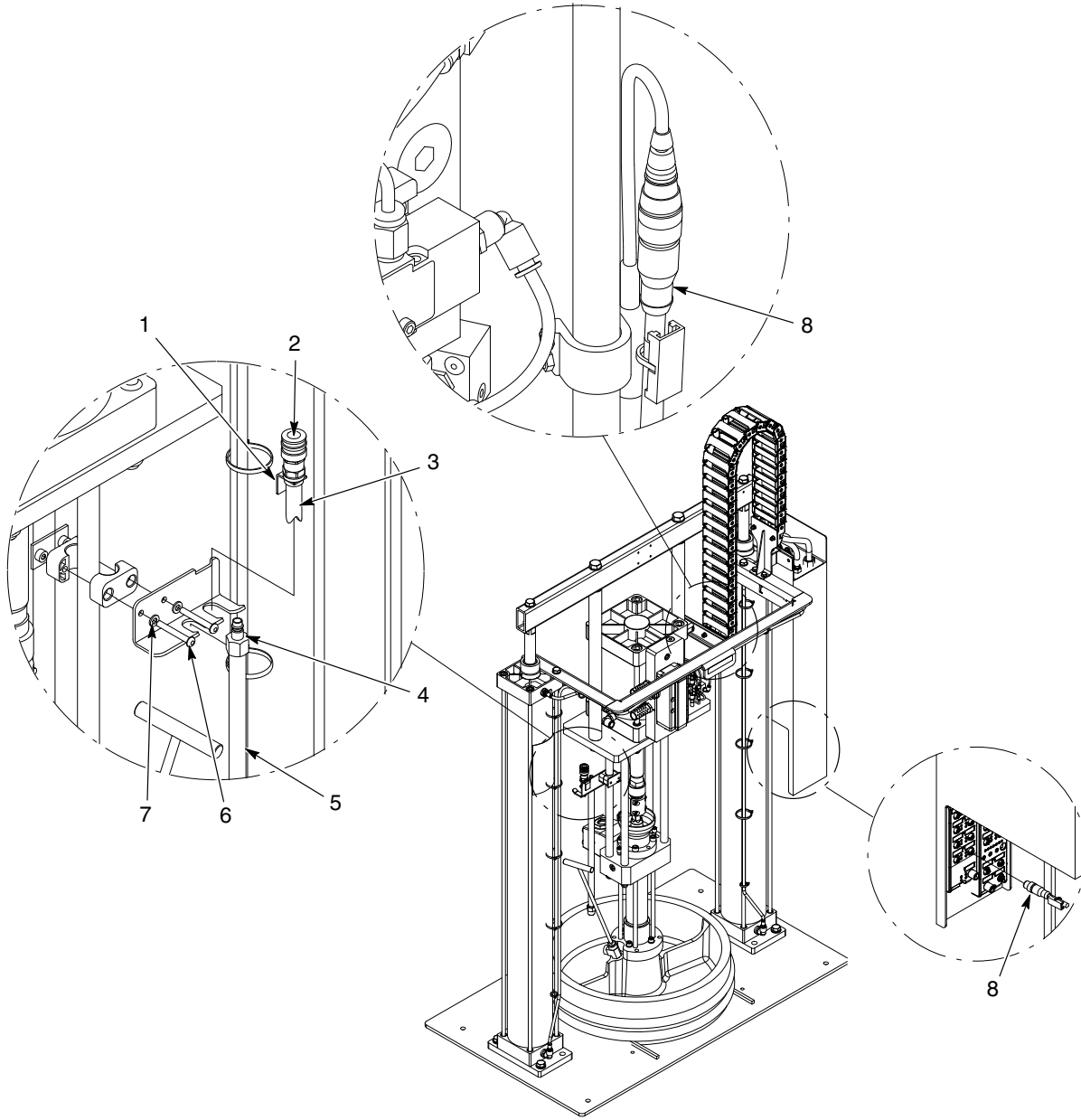
Şekil 10 SD3 hava motorlu küçük/büyük çerçeve hortum modülü, 24 Vdc (3/3)
