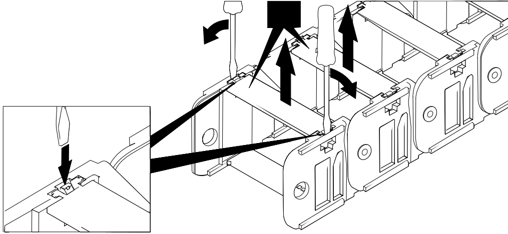
Şekil 2 Kablo zinciri
