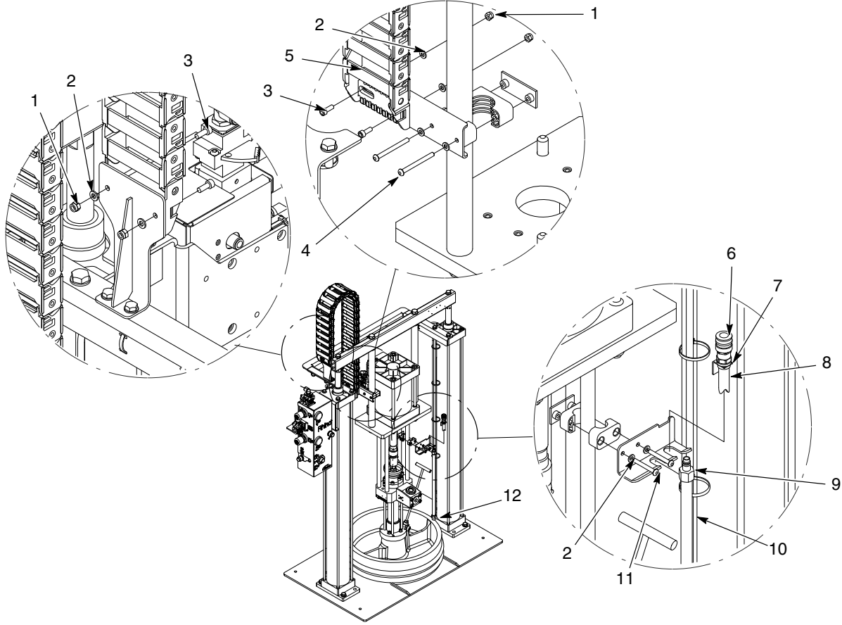
Şekil 24 SD2 hava motorlu küçük/büyük çerçeve hortum modülü, 5 galon ve 55 galon, pnömatik (1/2)
