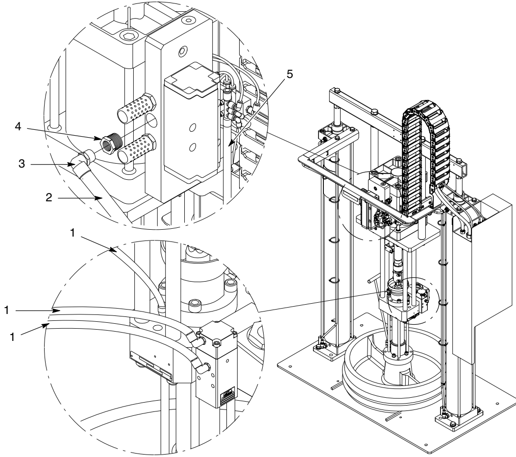
Şekil 12 SD2 hava motorlu küçük/büyük çerçeve hortum modülü, 24 Vdc (2/3)
