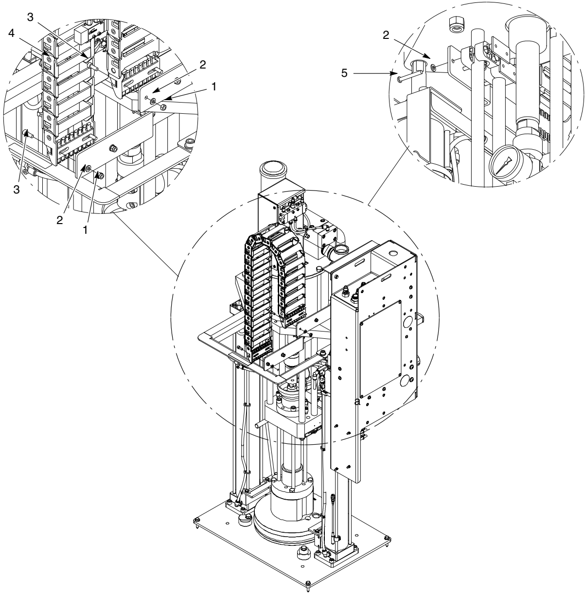
Şekil 7 SD2 hava motorlu DP çerçeve hortum modülü, 24 Vdc (2/2)
