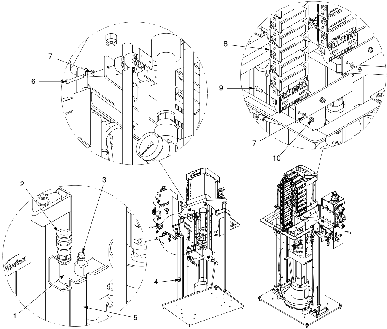
Şekil 18 SD3 hava motorlu DP çerçeve hortum modülü, pnömatik (1/2)
