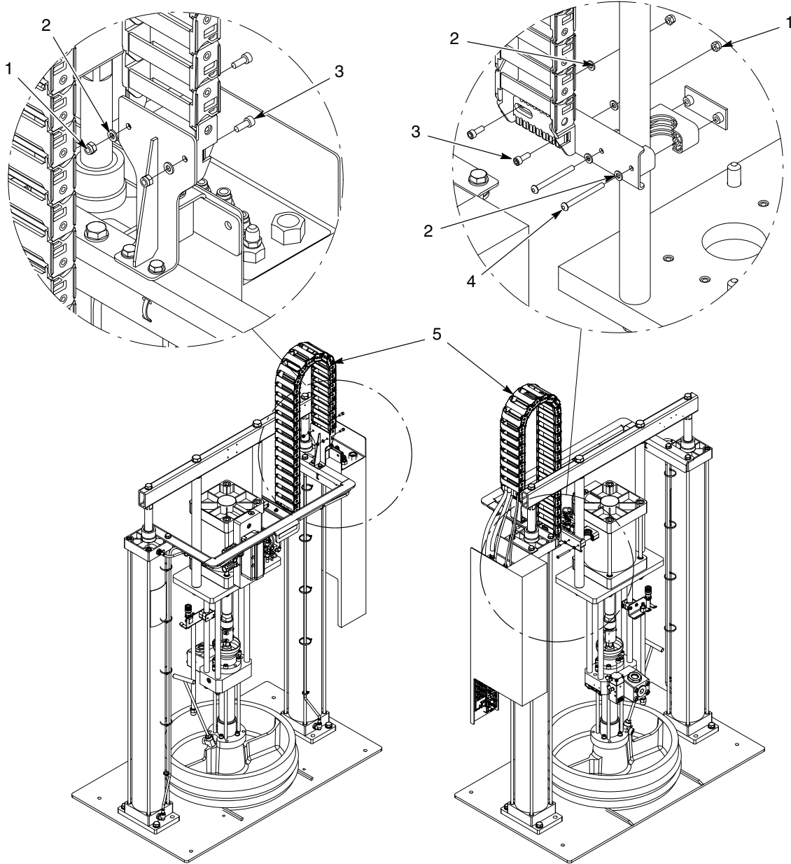
Şekil 8 SD3 hava motorlu küçük/büyük çerçeve hortum modülü, 24 Vdc (1/3)
