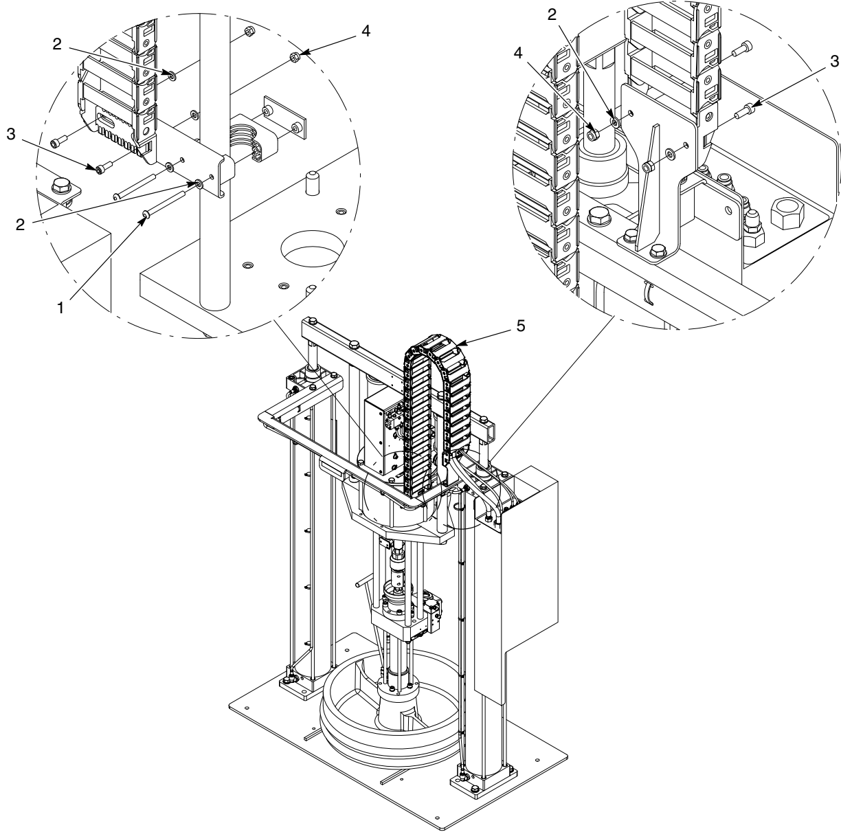
Şekil 16 SD2 hava motorlu küçük/büyük çerçeve hortum modülü, MT, 24 Vdc (1/2)
