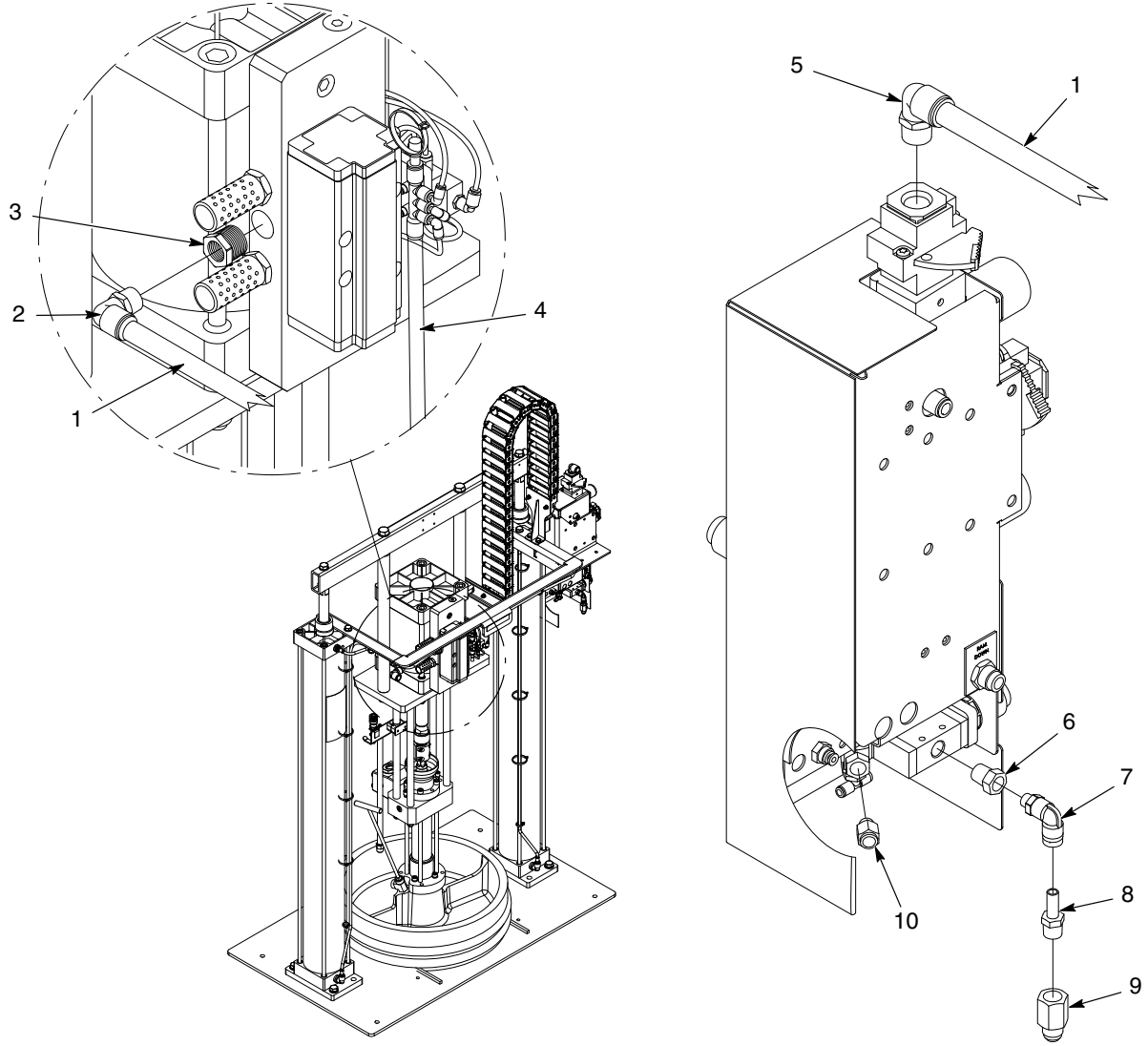
Şekil 23 SD3 hava motorlu küçük/büyük çerçeve hortum modülü, 55 galon, pnömatrik (2/2)
