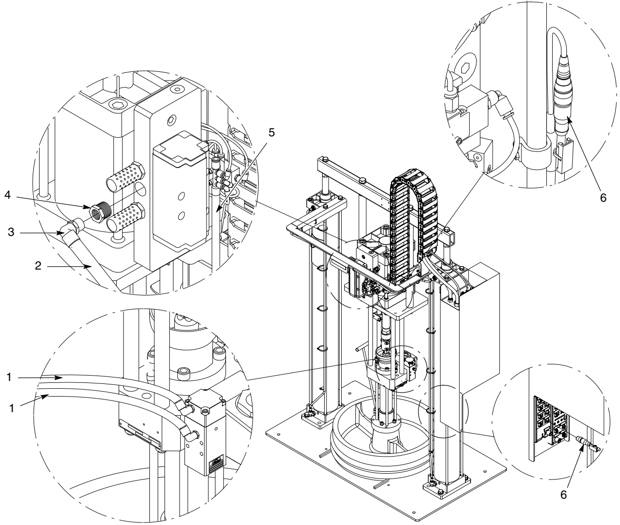
Şekil 15 SD3 hava motorlu küçük/büyük çerçeve hortum modülü, MT, 24 Vdc (2/2)
