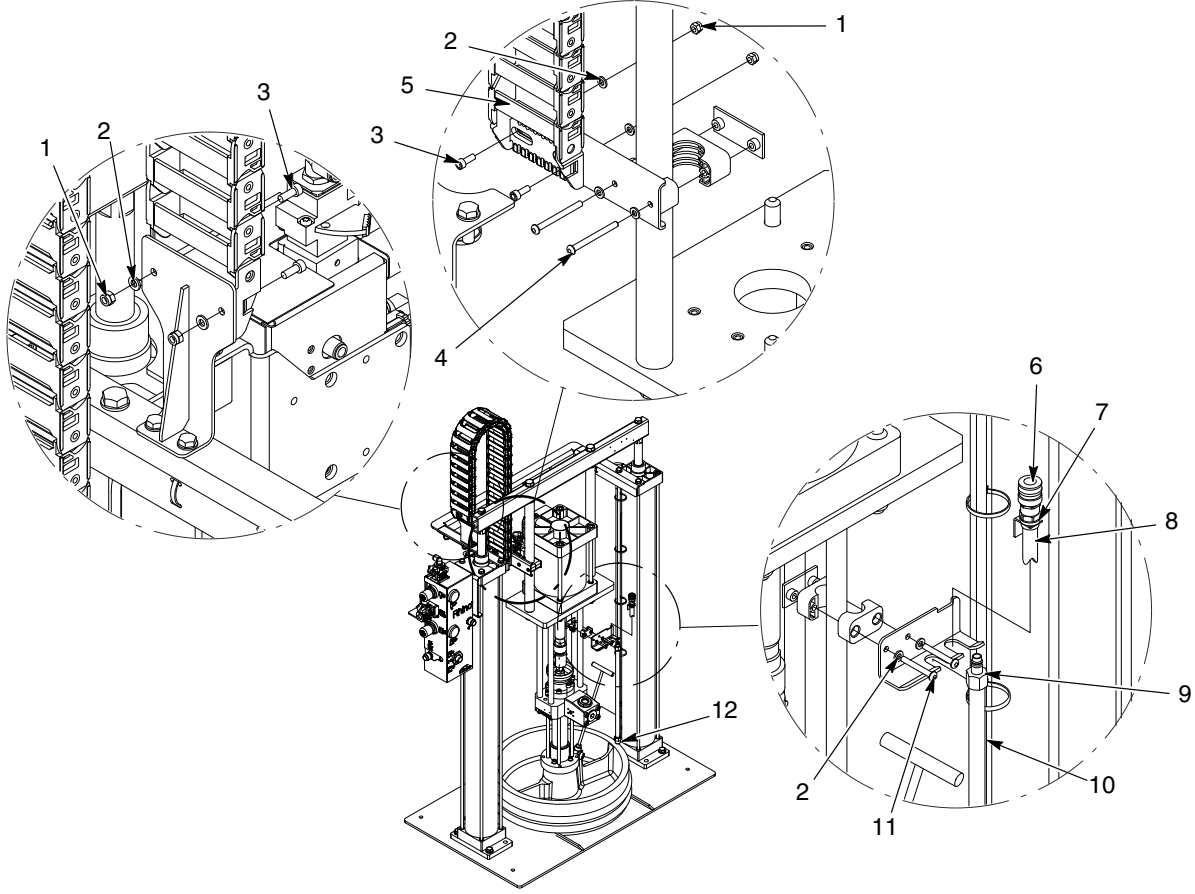
Şekil 22 SD3 hava motorlu küçük/büyük çerçeve hortum modülü, 55 galon, pnömatik (1/2)
