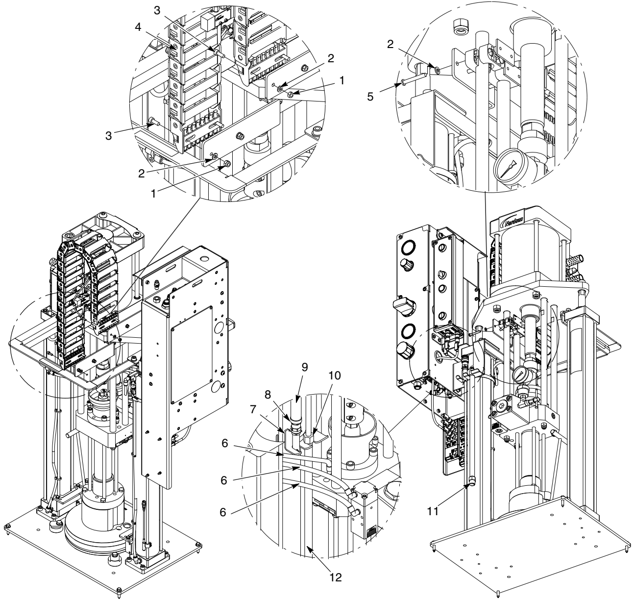
Şekil 5 SD3 hava motorlu DP çerçeve hortum modülü, 24 Vdc (2/2)
