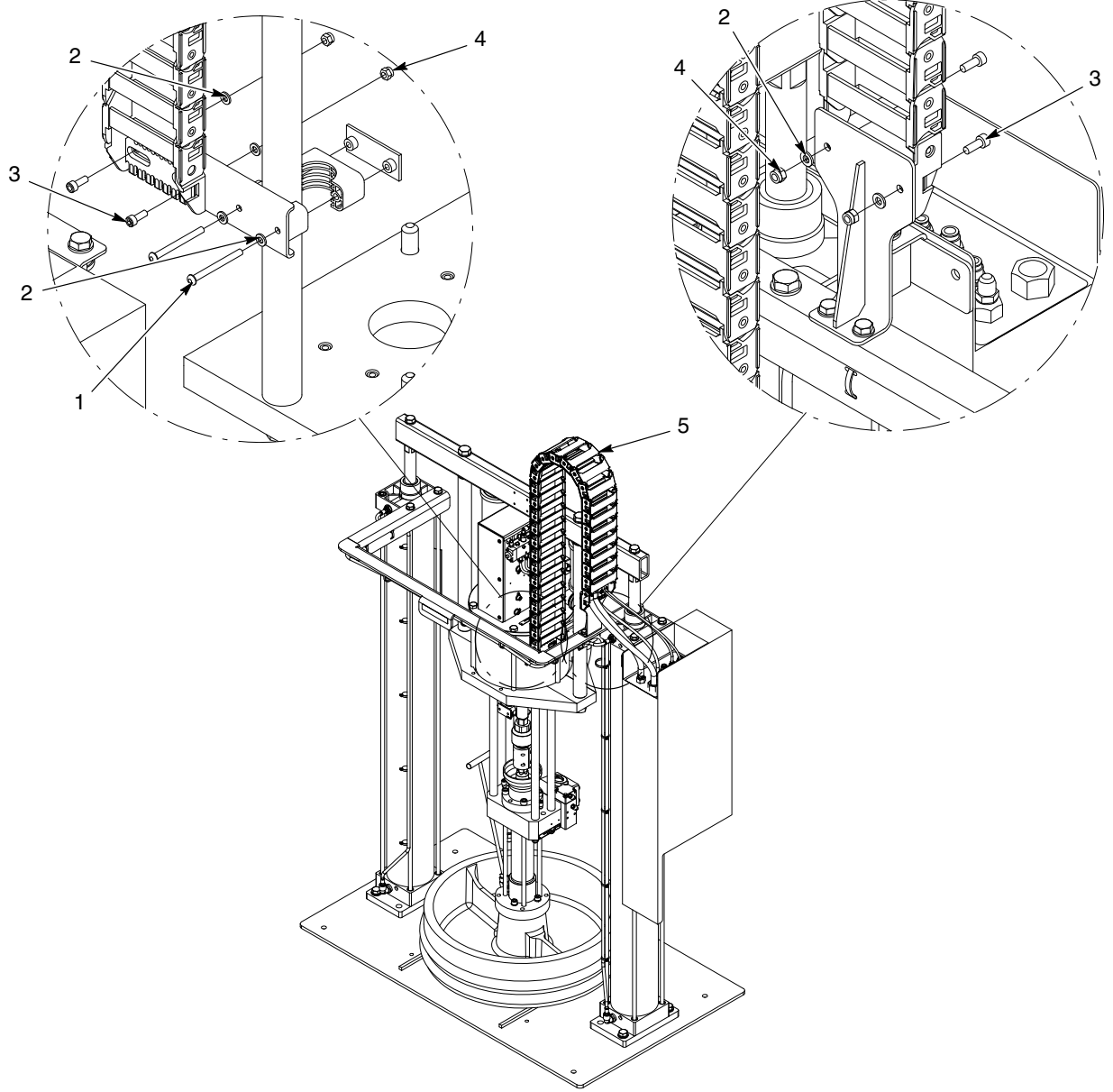
Şekil 11 SD2 hava motorlu küçük/büyük çerçeve hortum modülü, 24 Vdc (1/3)
