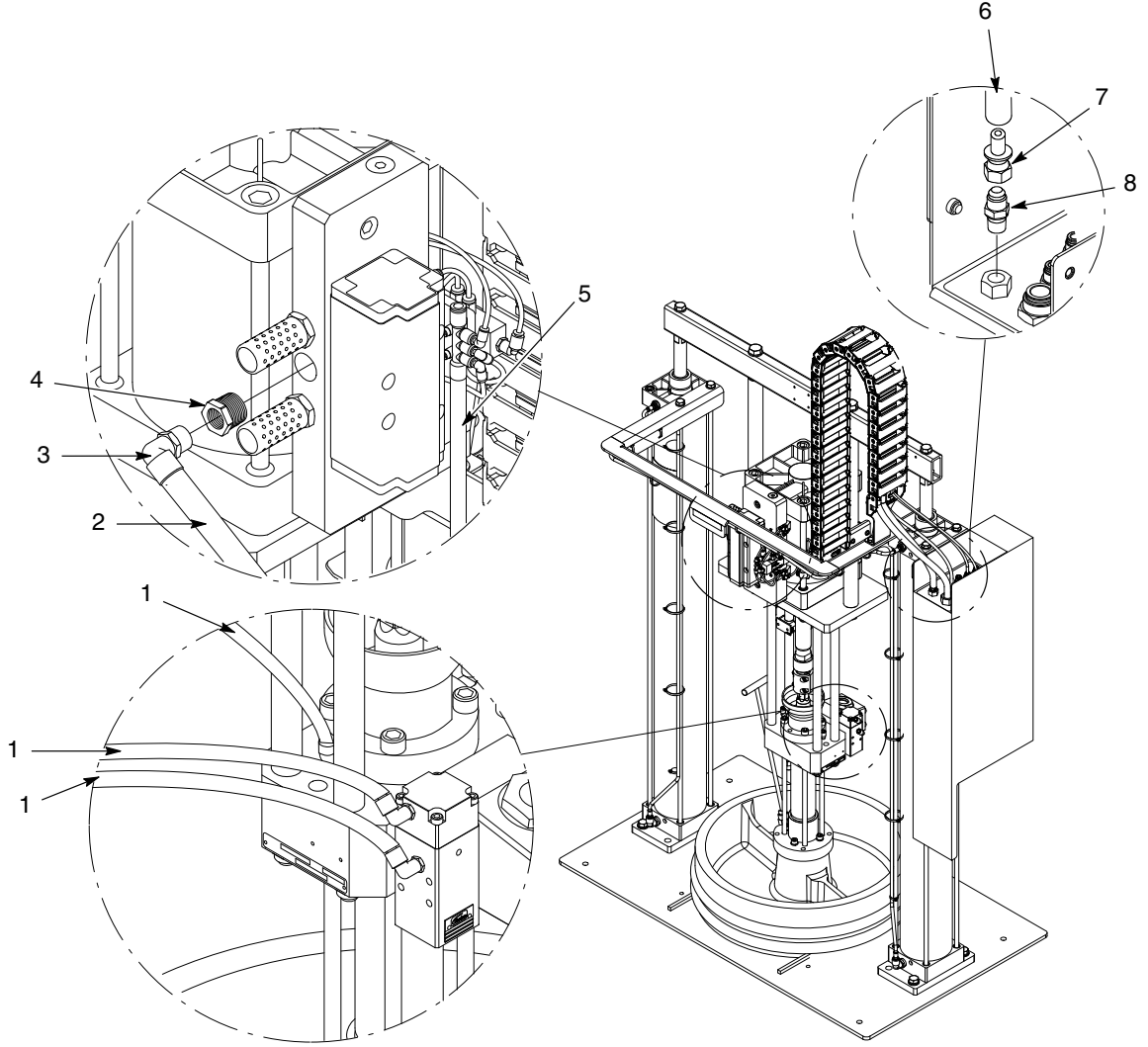
Şekil 9 SD3 hava motorlu küçük/büyük çerçeve hortum modülü, 24 Vdc (2/3)
