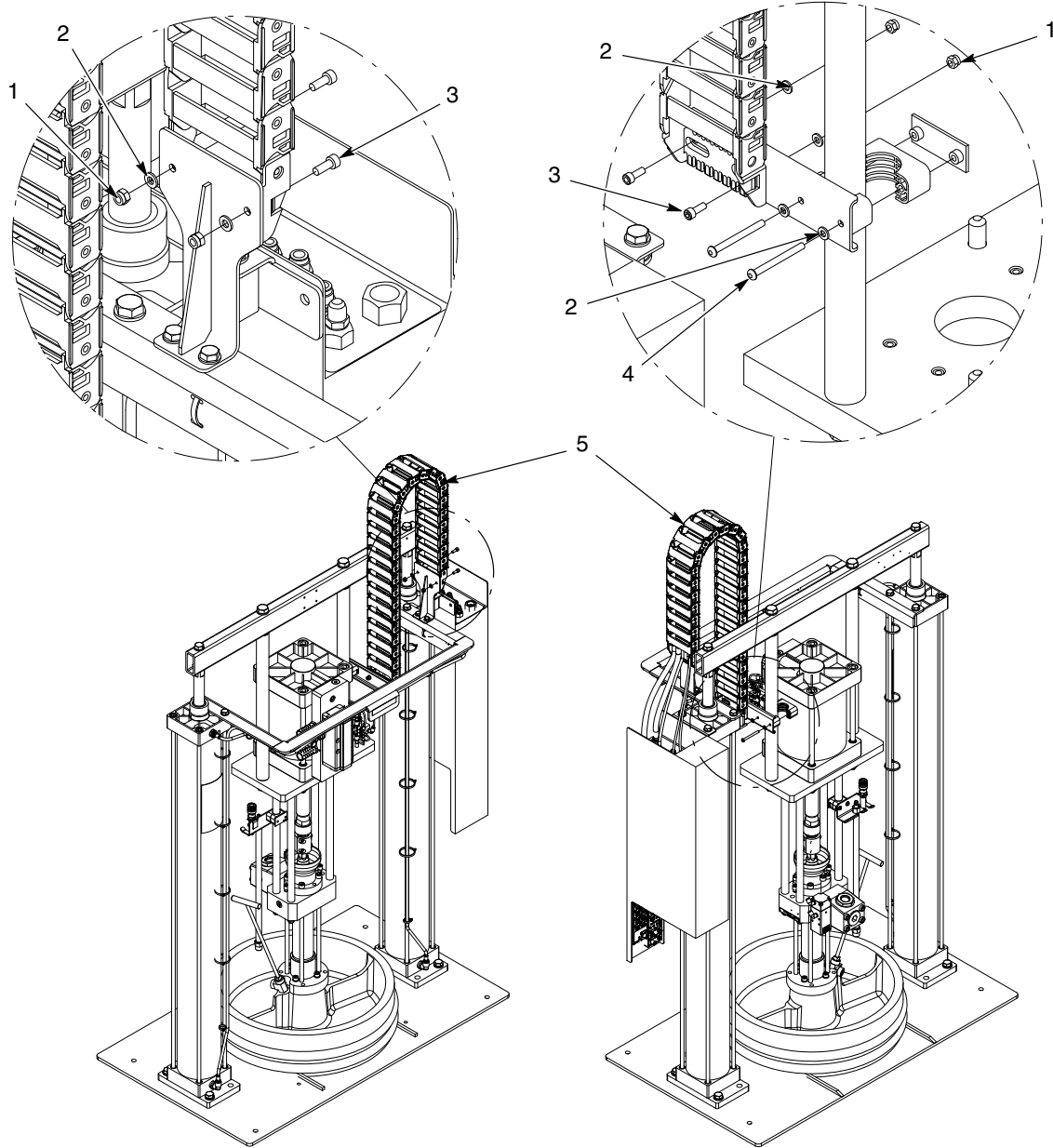
Şekil 14 SD3 hava motorlu küçük/büyük çerçeve hortum modülü, MT, 24 Vdc (1/2)
