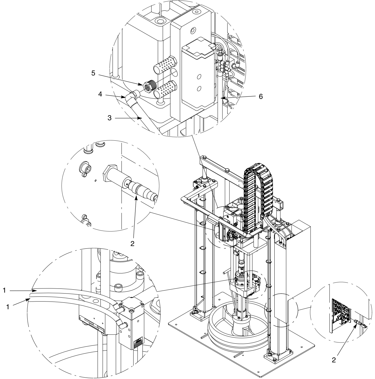
Şekil 17 SD2 hava motorlu küçük/büyük çerçeve hortum modülü, MT, 24 Vdc (2/2)
