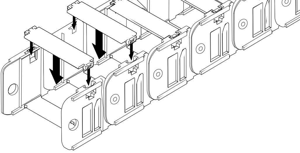
Şekil 3 Kablo zinciri
