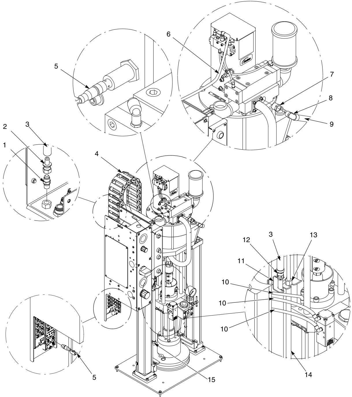
Şekil 6 SD2 hava motorlu DP çerçeve hortum modülü, 24 Vdc (1/2)
