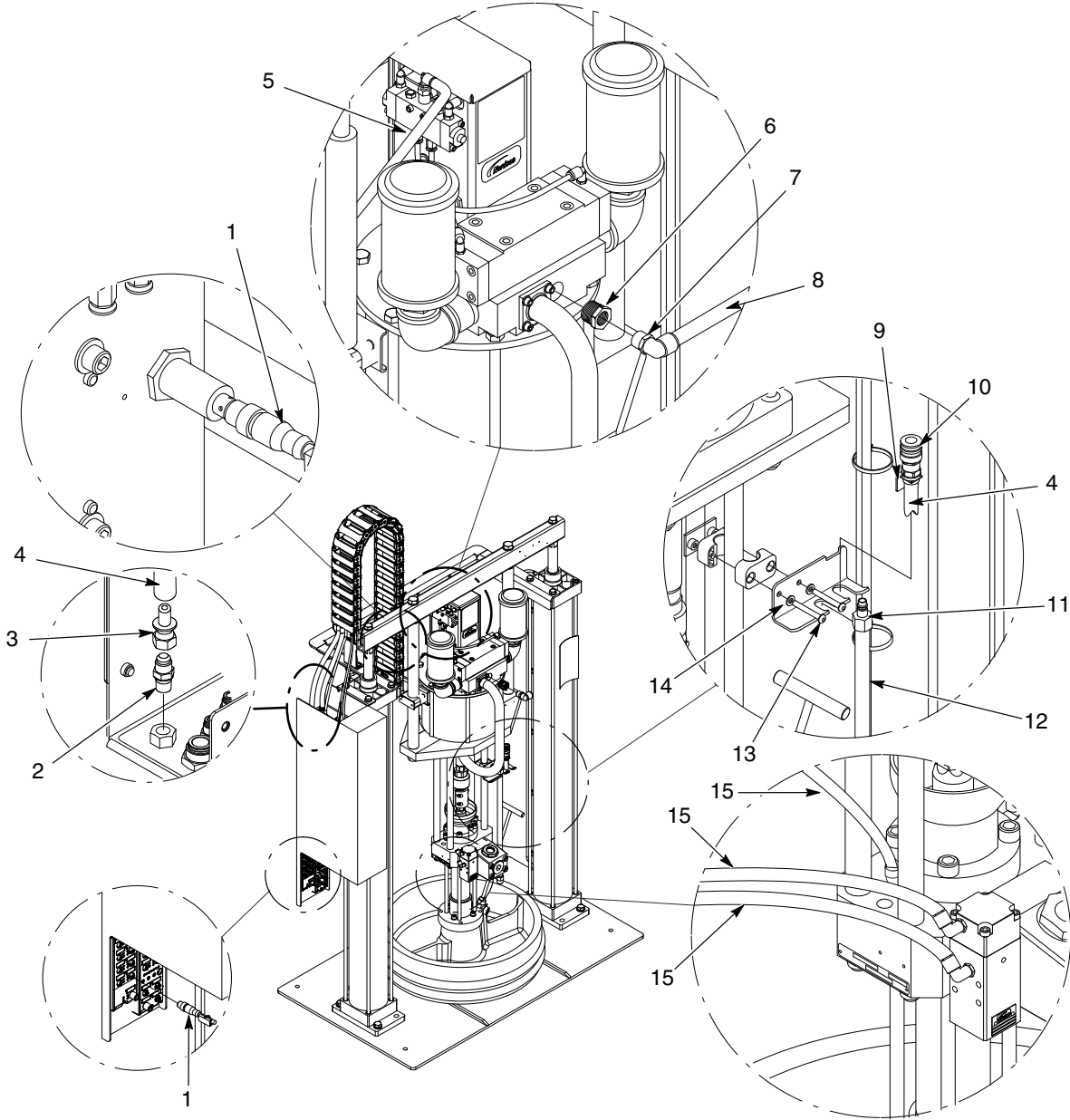
Şekil 13 SD2 hava motorlu küçük/büyük çerçeve hortum modülü, 24 Vdc (3/3)
