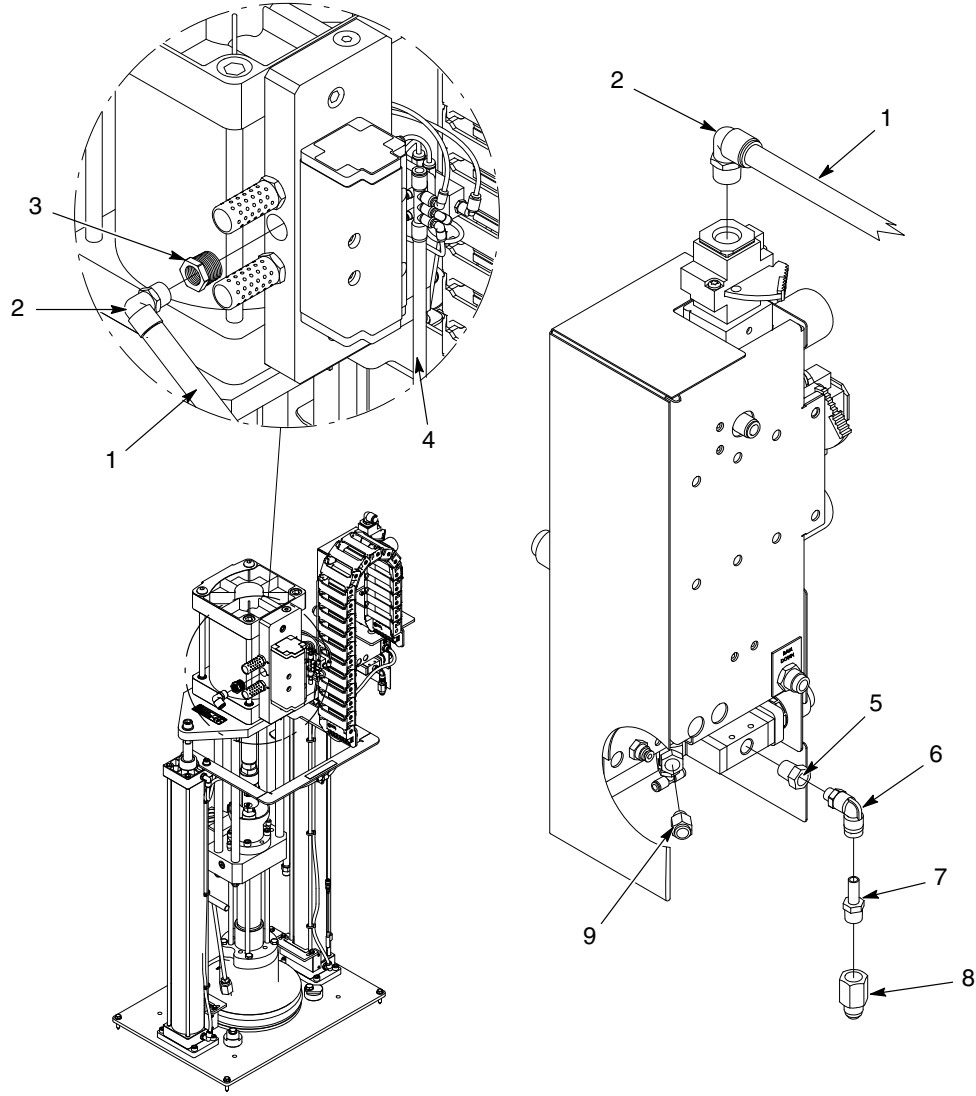
Şekil 19 SD3 hava motorlu DP çerçeve hortum modülü, pnömatik (2/2)
