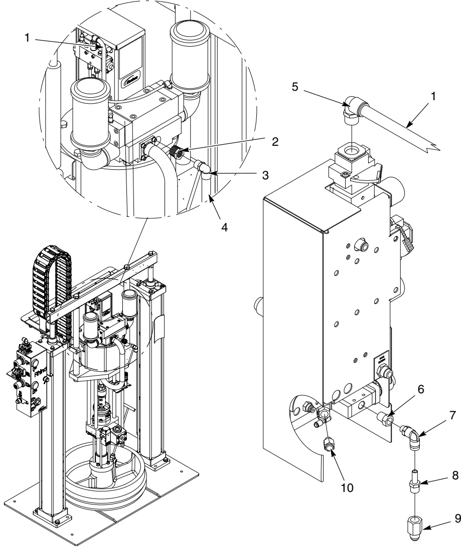
Şekil 25 SD2 hava motorlu küçük/büyük çerçeve hortum modülü, 5 galon ve 55 galon, pnömatik (2/2)
