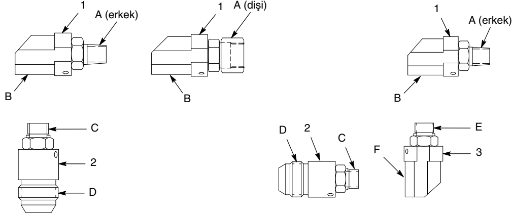
Şekil 1 Küçük döner tablalar - tipik kombinasyonlar
