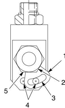
Şekil 4 Döner kilit anahtarı
