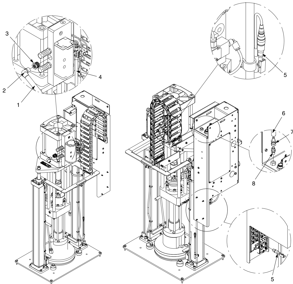
图 4 带 SD3 气动马达的 DP 框架胶管模块，24 Vdc (1/2)
