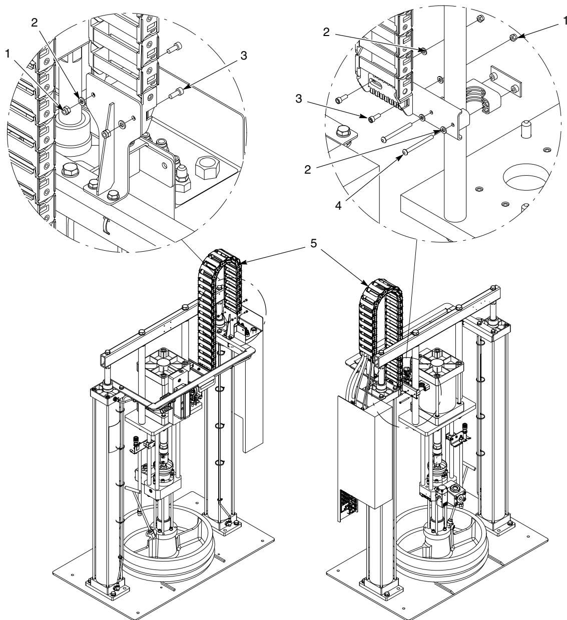
图 14 带 SD3 气动马达的小型/大型框架胶管模块, MT, 24 Vdc (1/2)
