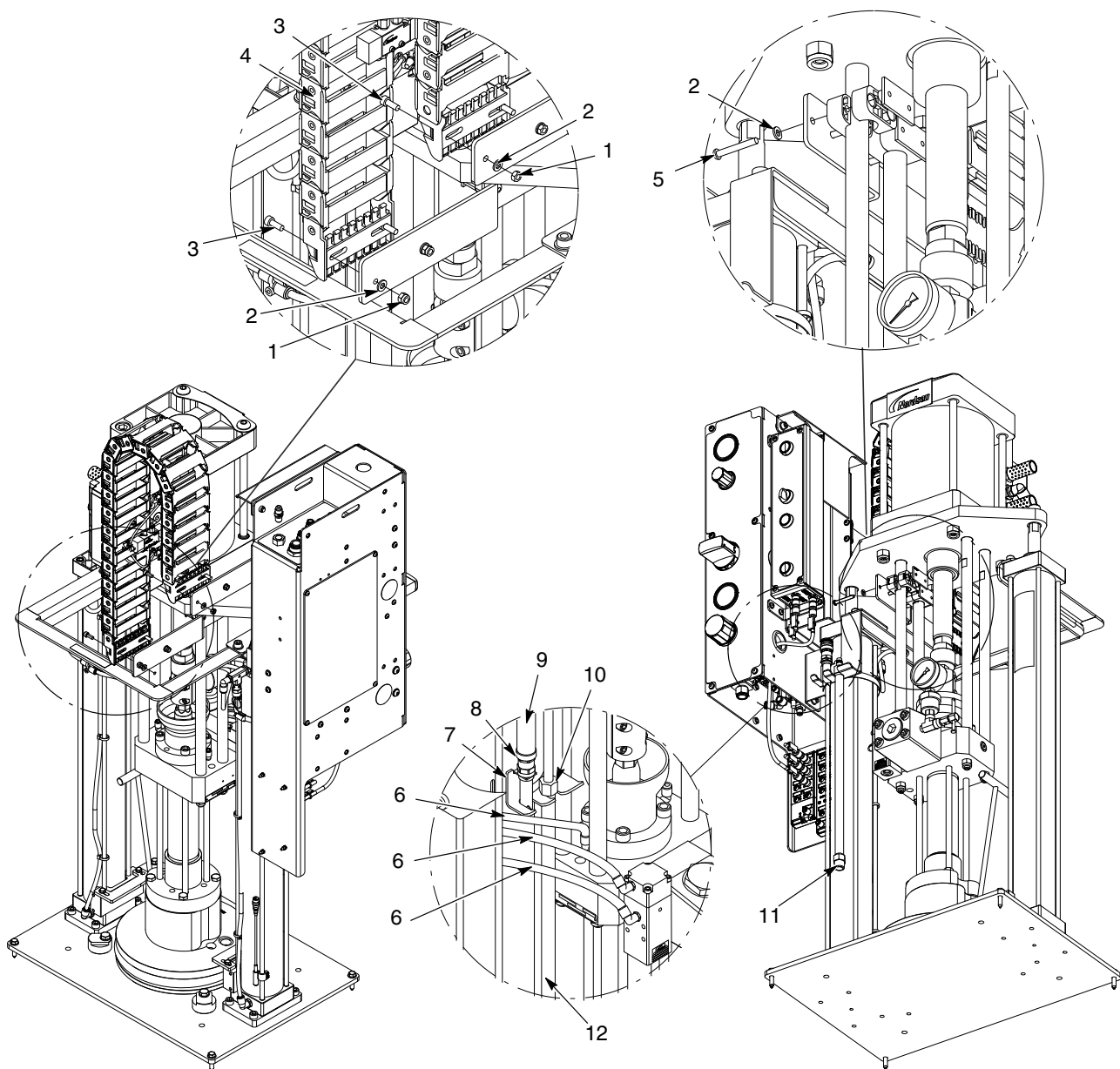
图 5 带 SD3 气动马达的 DP 框架胶管模块, 24 Vdc (2/2)
