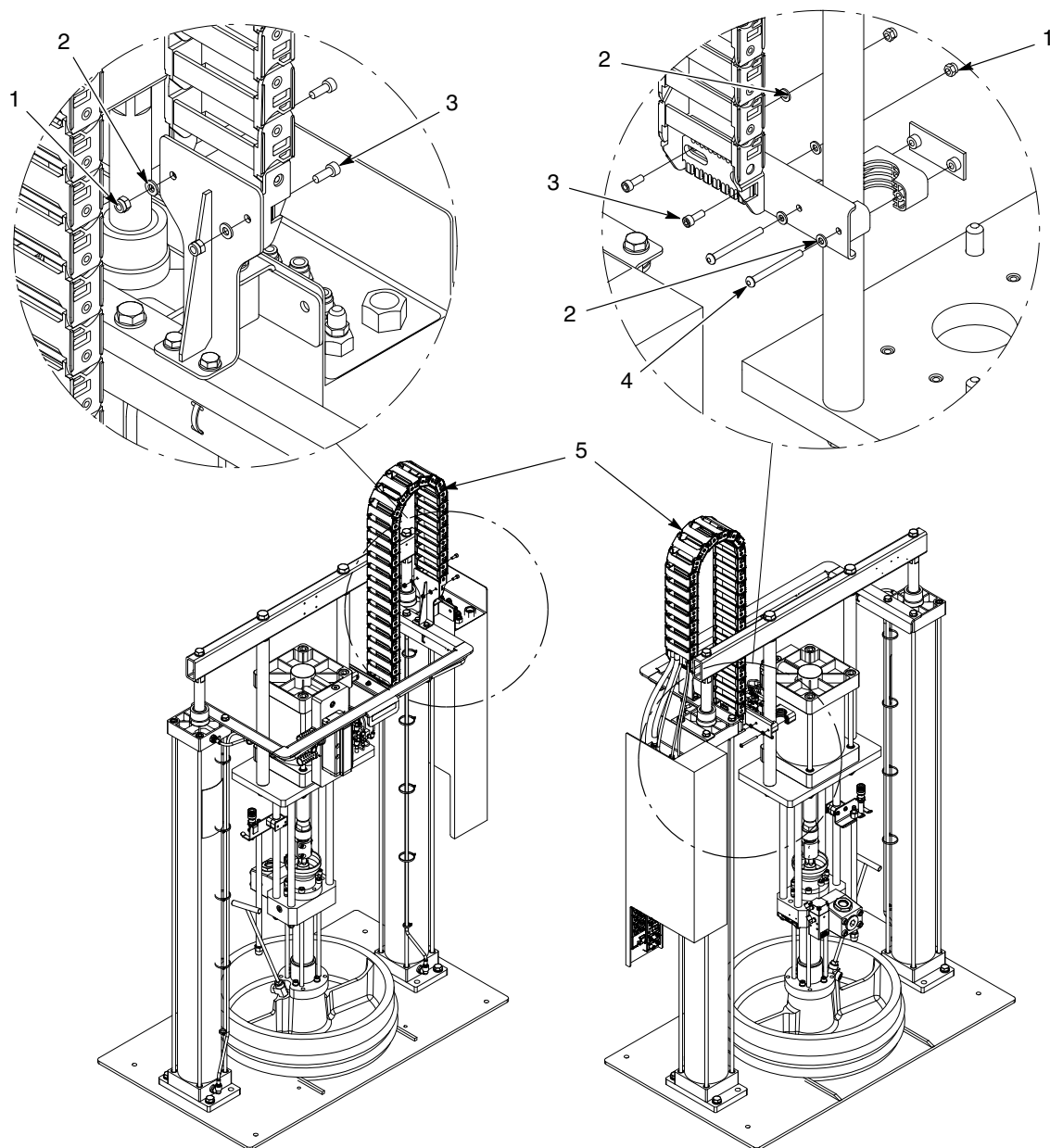
图 8 带 SD3 气动马达的小型/大型框架胶管模块, 24 Vdc (1/3)
