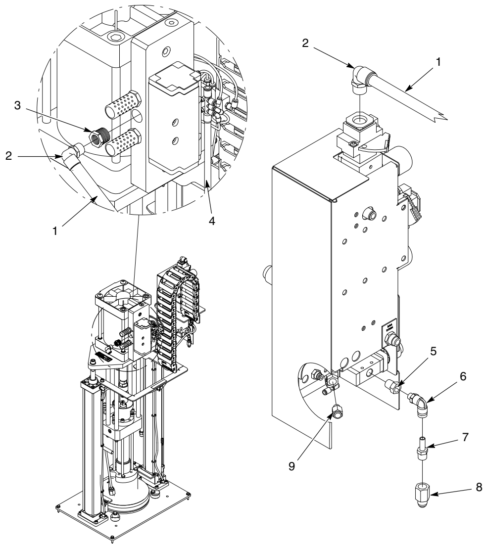
图 19 带 SD3 气动马达的 DP 框架胶管模块, 气动 (2/2)
