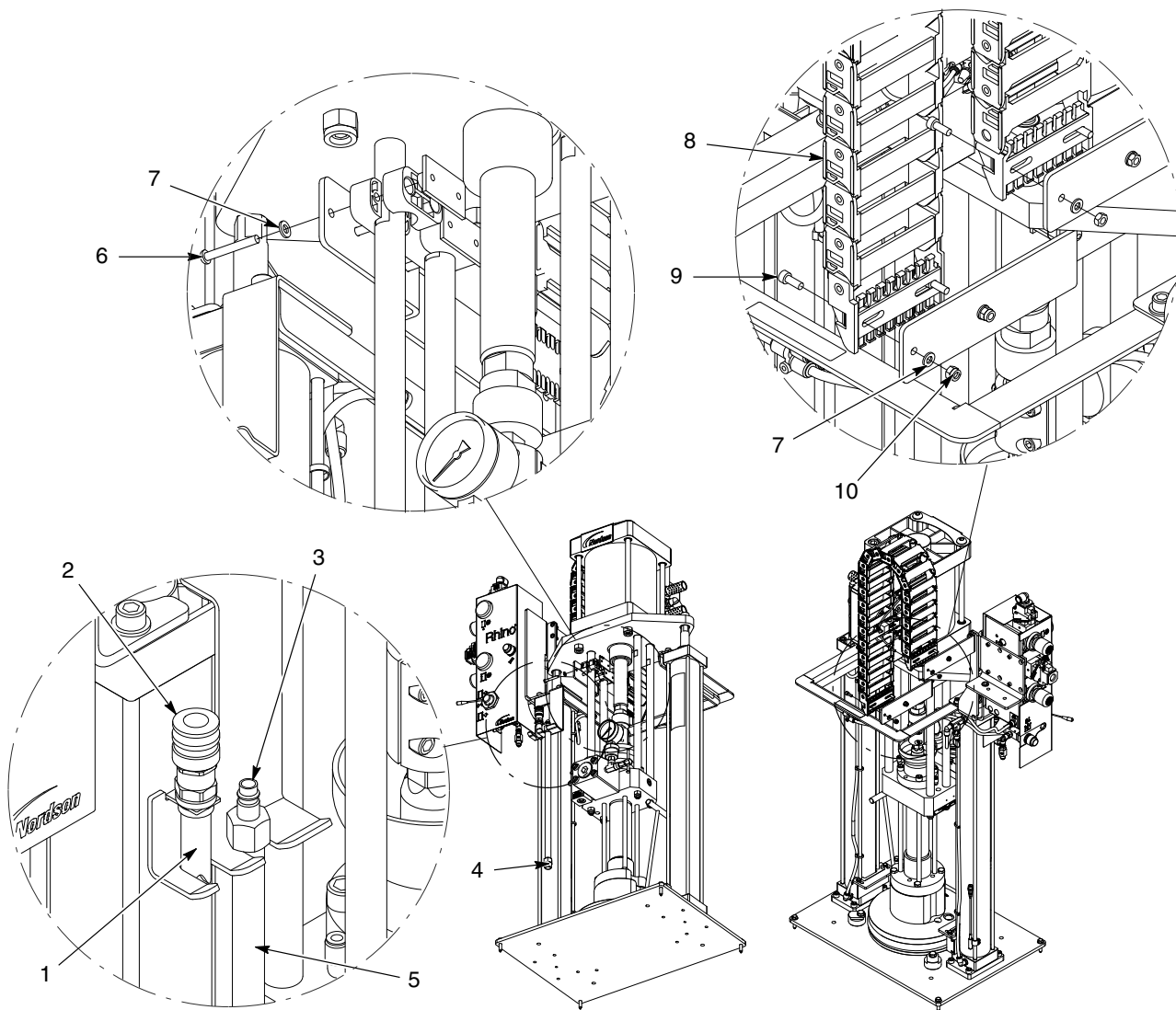
图 18 带 SD3 气动马达的 DP 框架胶管模块，气动 (1/2)
