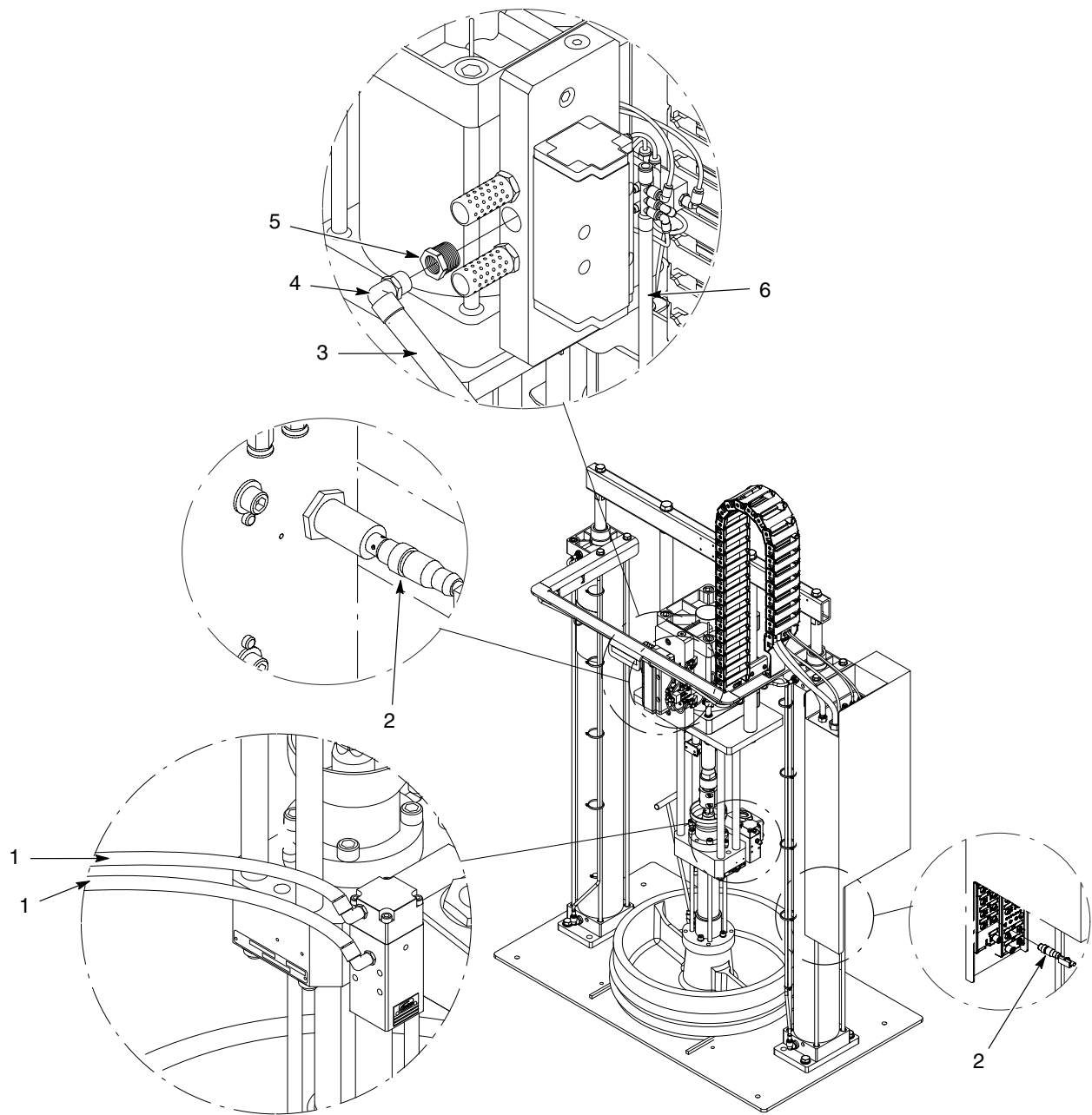
图 17 带 SD2 气动马达的小型/大型框架胶管模块, MT, 24 Vdc (2/2)
