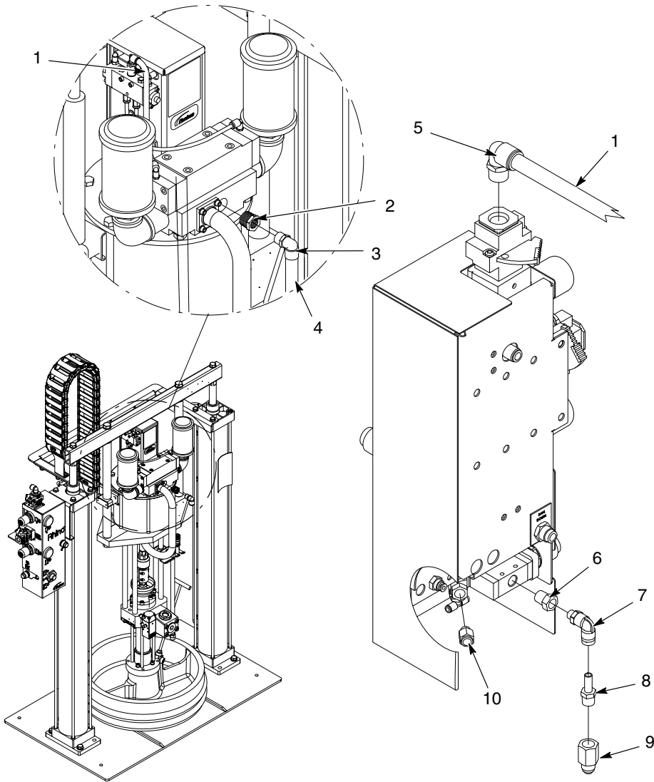
图 25 带 SD2 气动马达的小型/大型框架胶管模块，5 加仑和 55 加仑，气动 (2/2)
