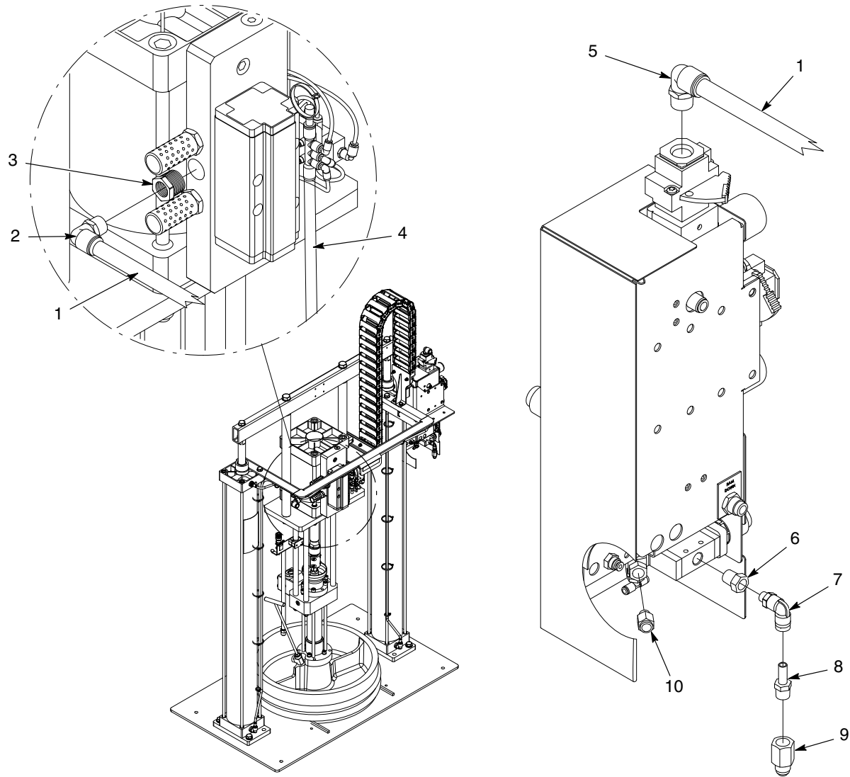
图 23 带 SD3 气动马达的小型/大型框架胶管模块, 55 加仑, 气动 (2/2)
