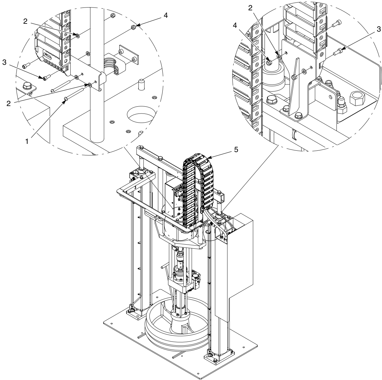
图 11 带 SD2 气动马达的小型/大型框架胶管模块，24 Vdc (1/3)
