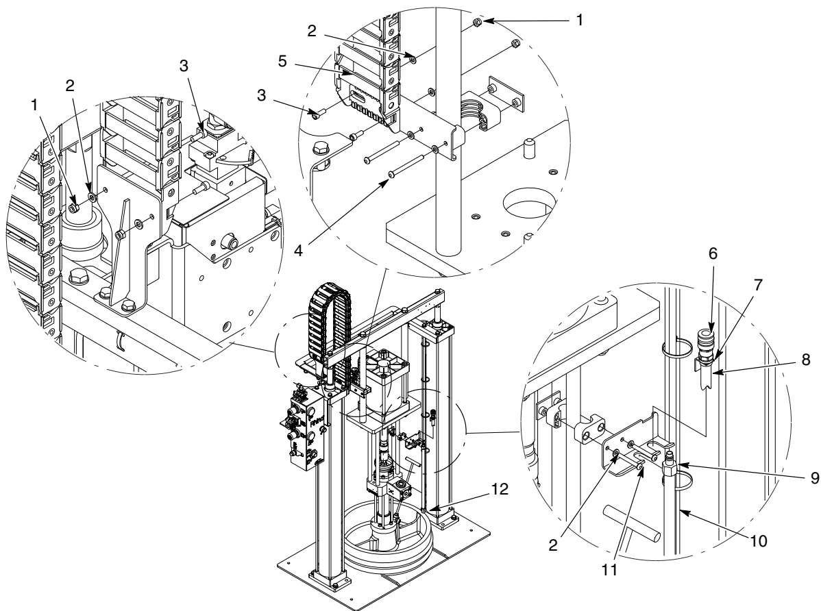
图 24 带 SD2 气动马达的小型/大型框架胶管模块, 5 加仑和 55 加仑, 气动 (1/2)
