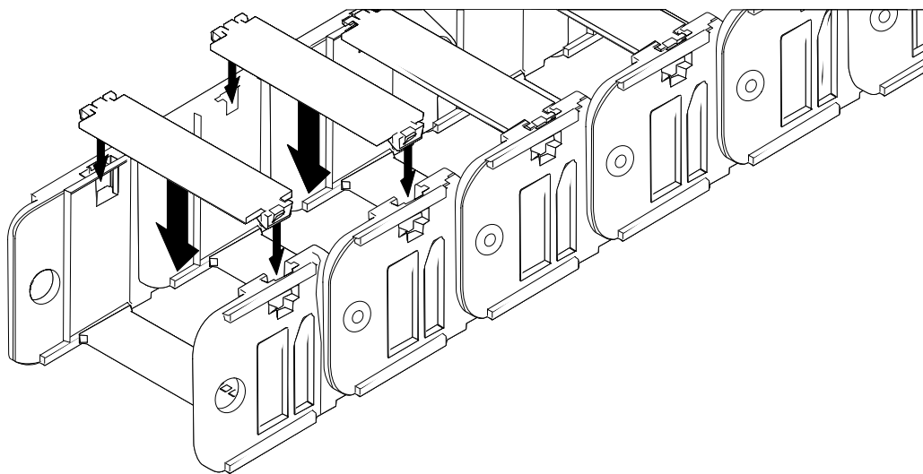
图 3 链轨
