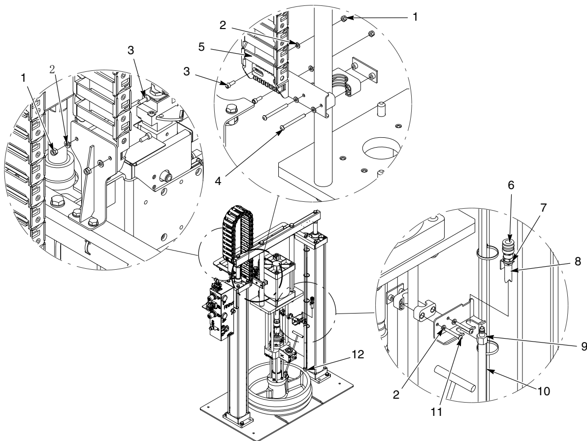
图 22 带 SD3 气动马达的小型/大型框架胶管模块, 55 加仑, 气动 (1/2)
