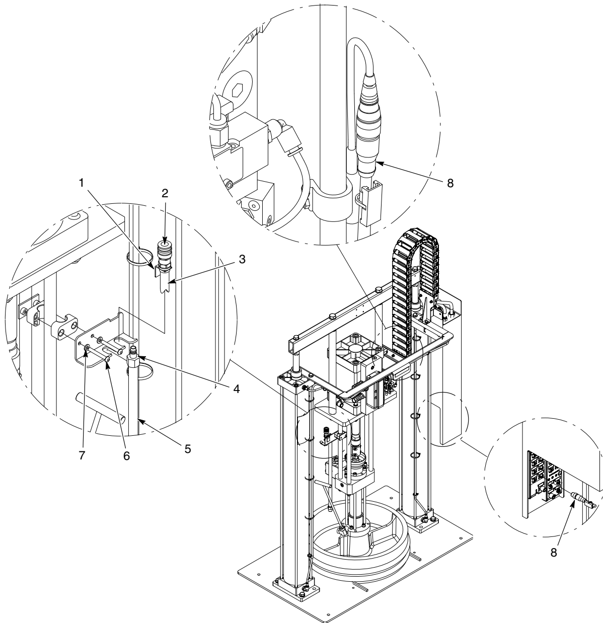
图 10 带 SD3 气动马达的小型/大型框架胶管模块, 24 Vdc (3/3)
