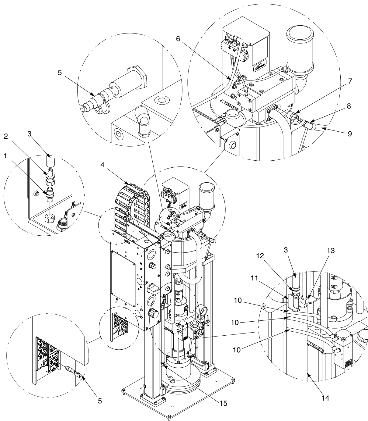
图 6 带 SD2 气动马达的 DP 框架胶管模块, 24 Vdc (1/2)
