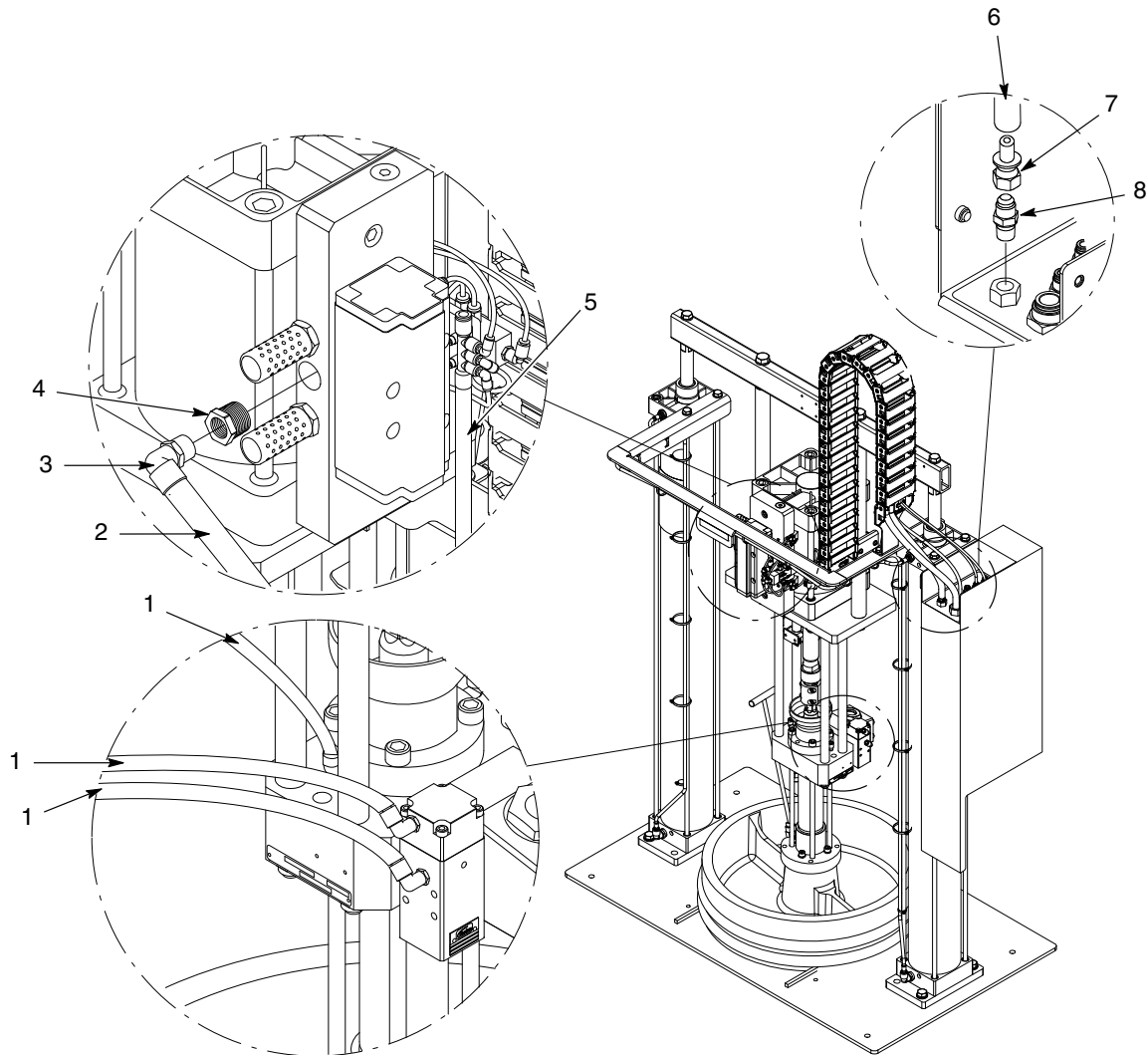
图 9 带 SD3 气动马达的小型/大型框架胶管模块, 24 Vdc (2/3)
