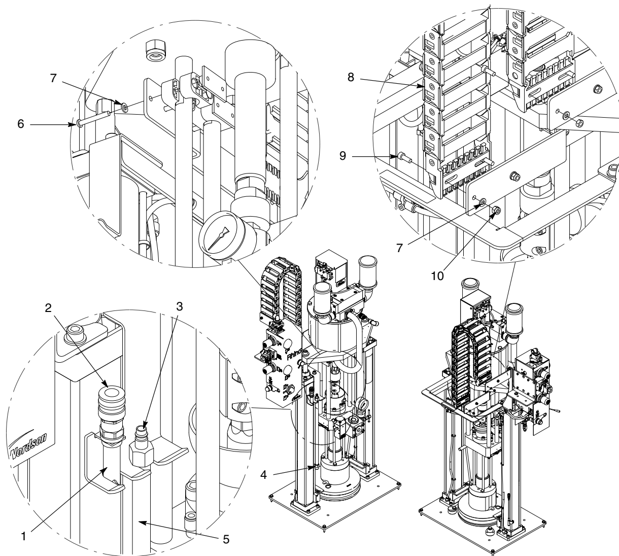
图 20 带 SD2 气动马达的 DP 框架胶管模块，气动 (1/2)
