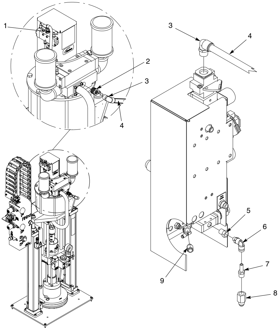
图 21 带 SD2 气动马达的 DP 框架胶管模块，气动（2/2）
