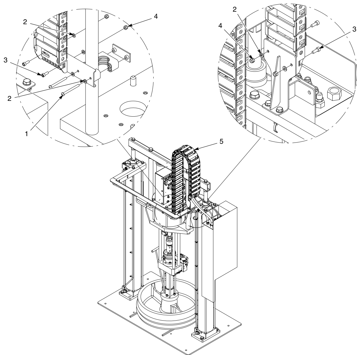
图 16 带 SD2 气动马达的小型/大型框架胶管模块, MT, 24 Vdc (1/2)
