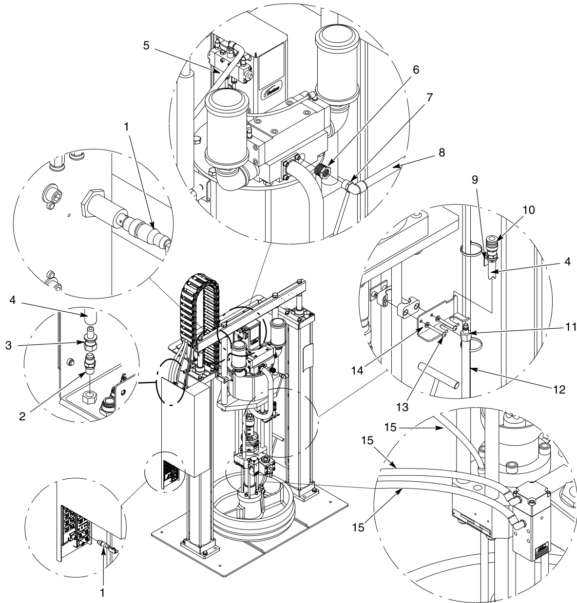
图 13 带 SD2 气动马达的小型/大型框架胶管模块，24 Vdc (3/3)
