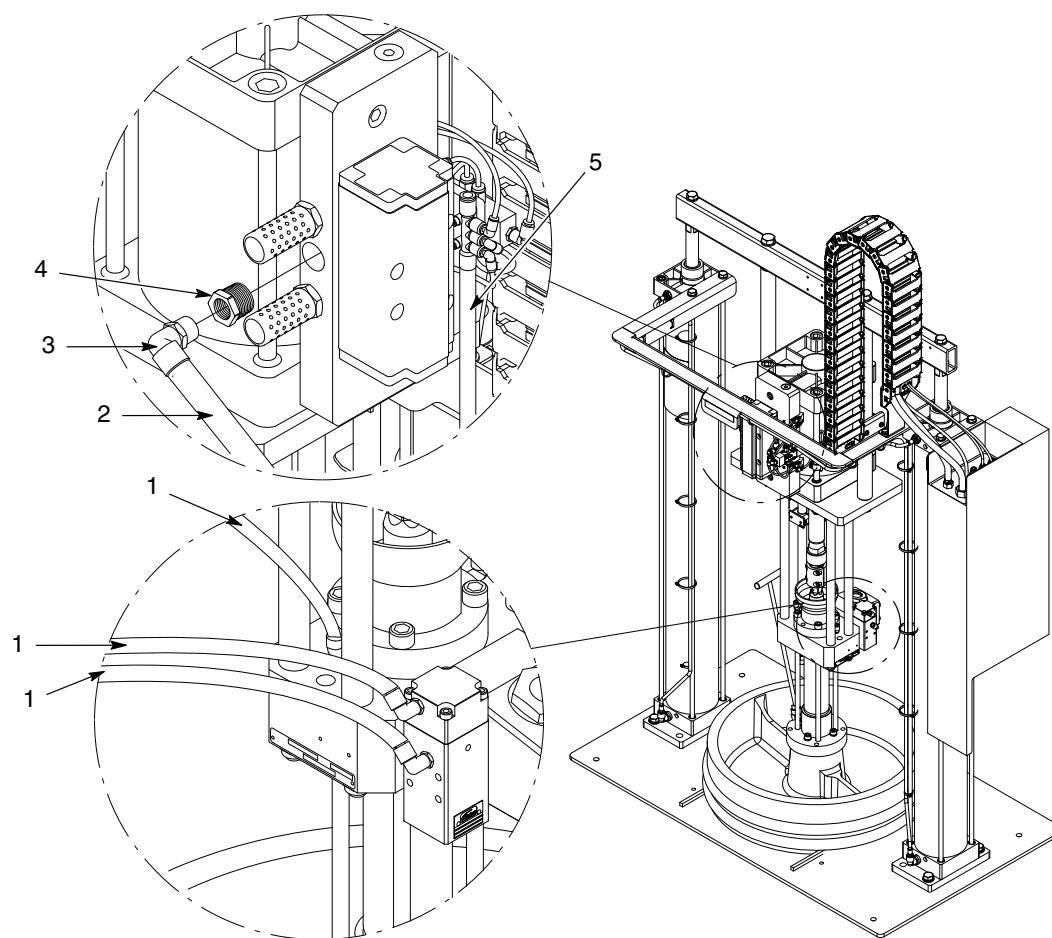
图 12 带 SD2 气动马达的小型/大型框架胶管模块, 24 Vdc (2/3)
