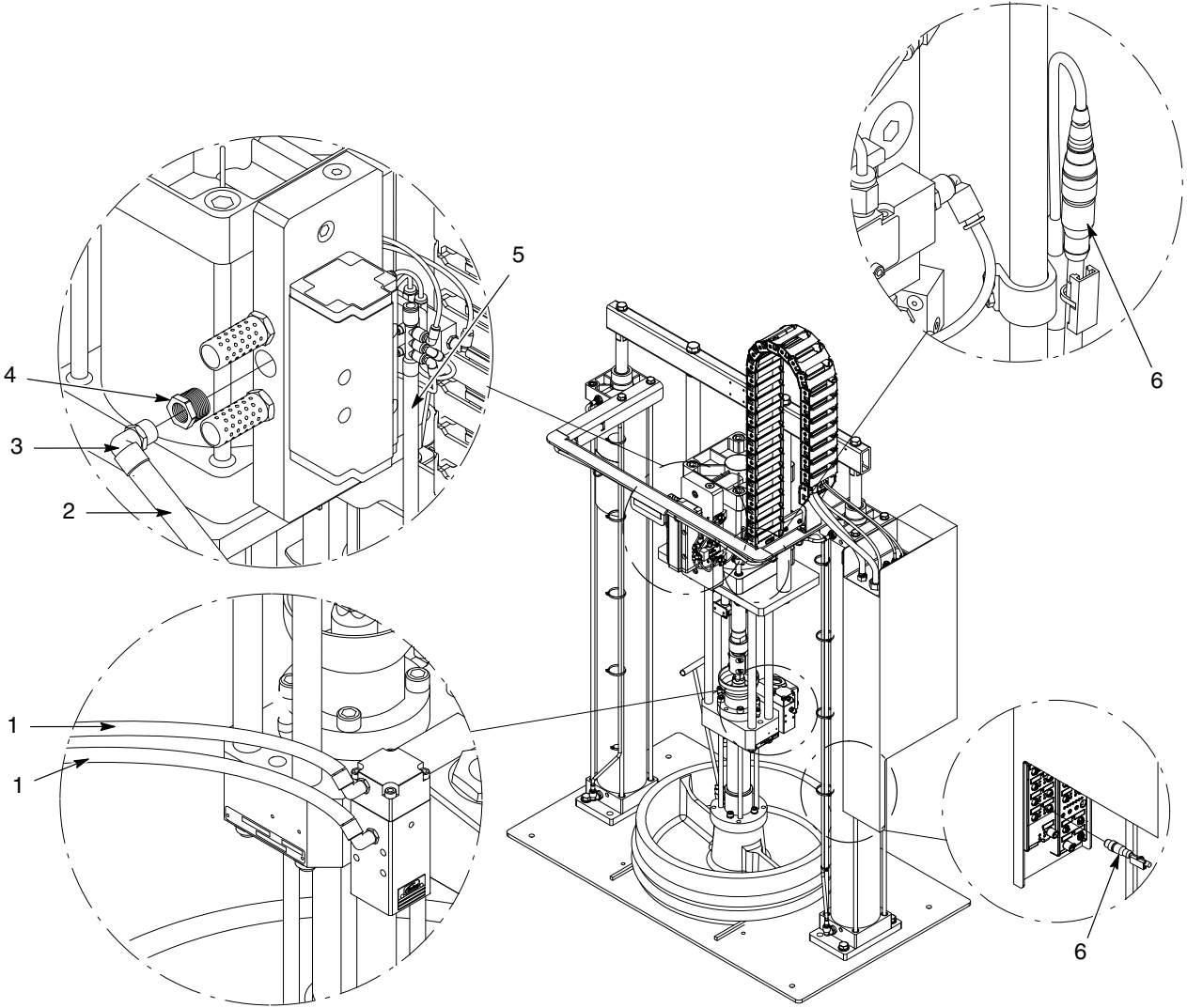
图 15 带 SD3 气动马达的小型/大型框架胶管模块，MT，24 Vdc (2/2)
