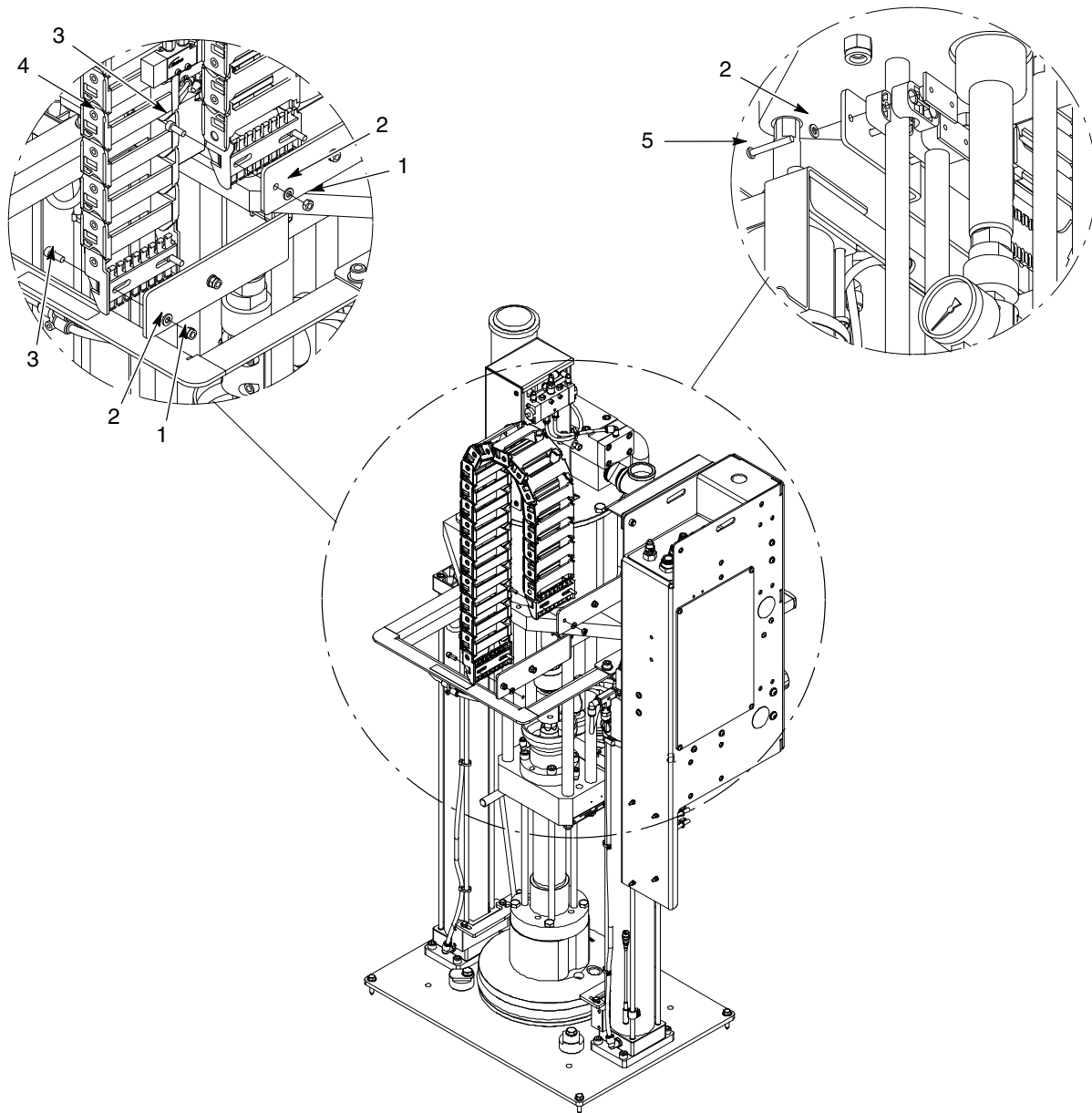
图 7 带 SD2 气动马达的 DP 框架胶管模块，24 Vdc (2/2)
